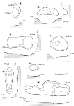
图46 土坑平面图
