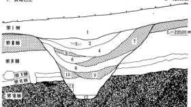
空堀SD2断面図
