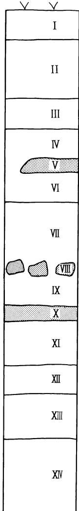
第4図 土層柱状図
