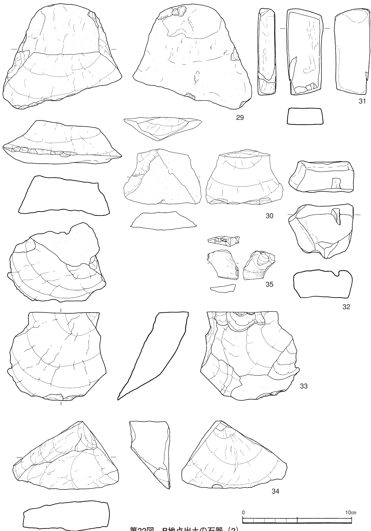
第22図 B地点出土の石器 (2)
