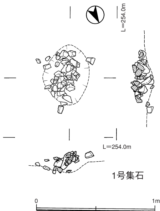
第95図 Ⅳ遺跡縄文時代前期以降の集石
