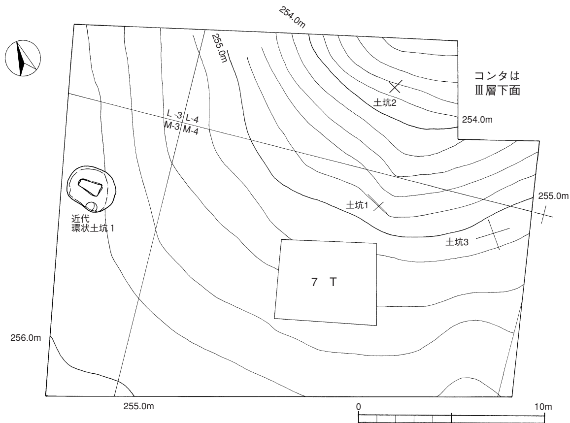
第11図 A地点遺構配置図
