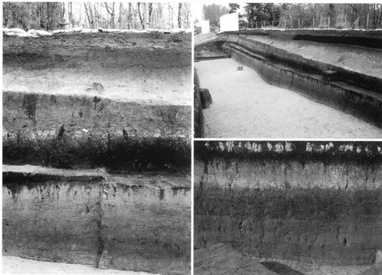
土層
