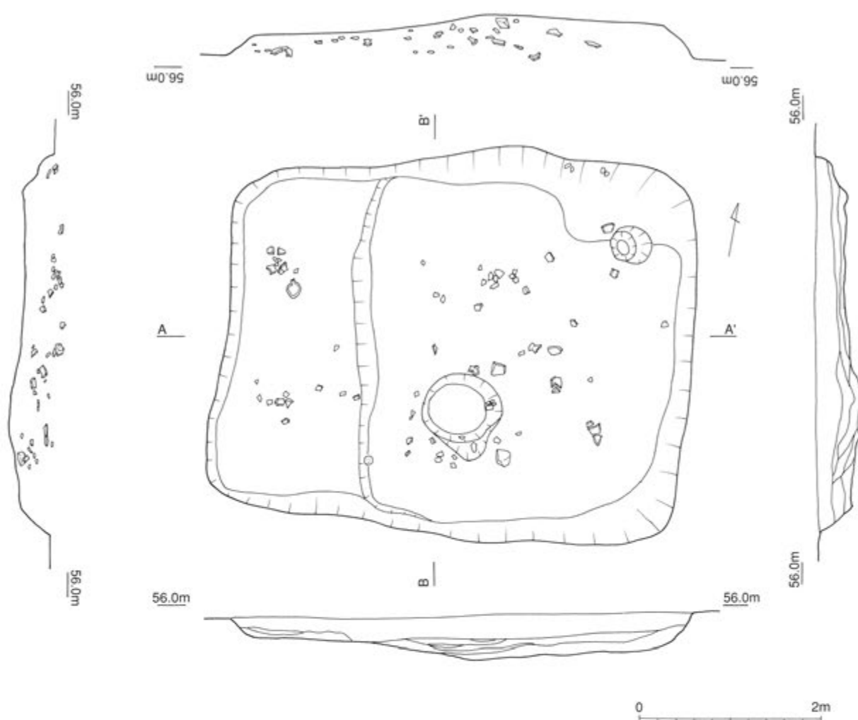
第101図 6号住居跡
