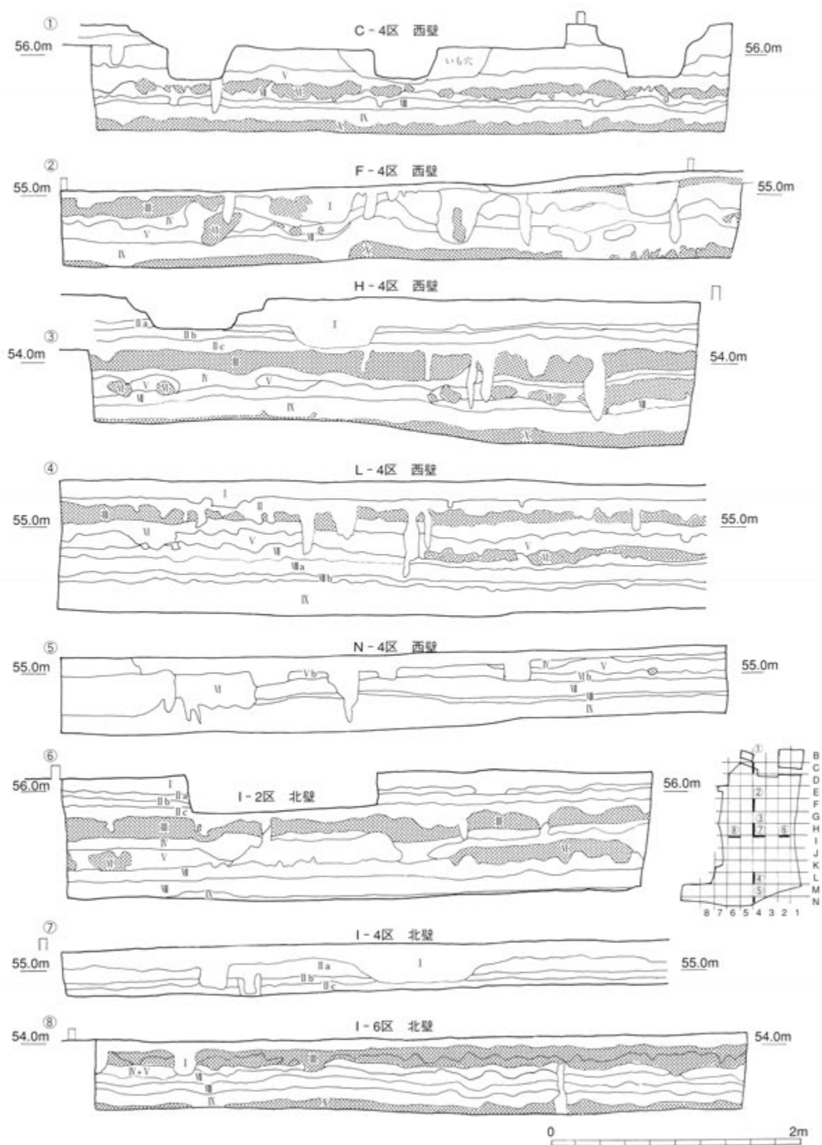
第5図 土層図3
