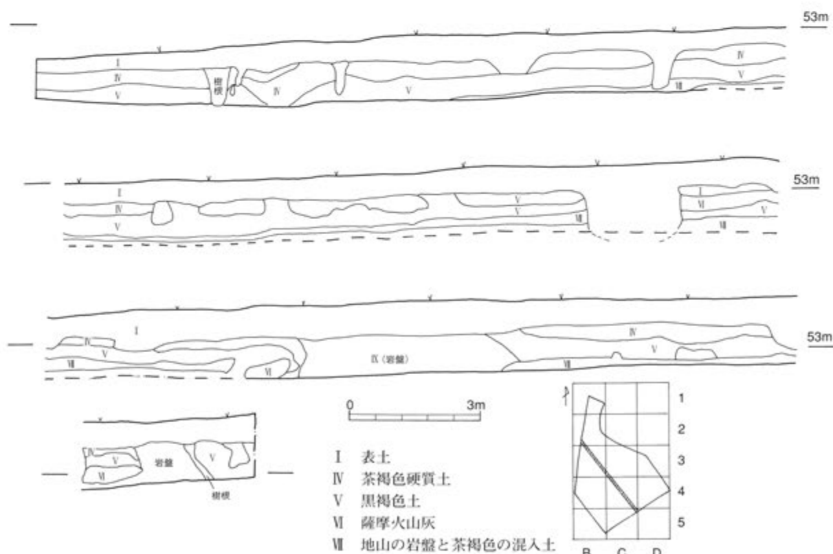
第2図 土層図
