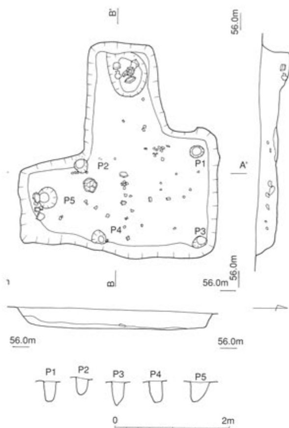
第99図 5号住居跡
