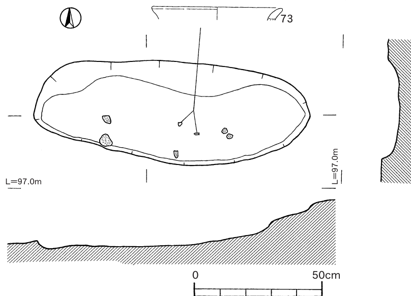
第29图 土坑(3)
