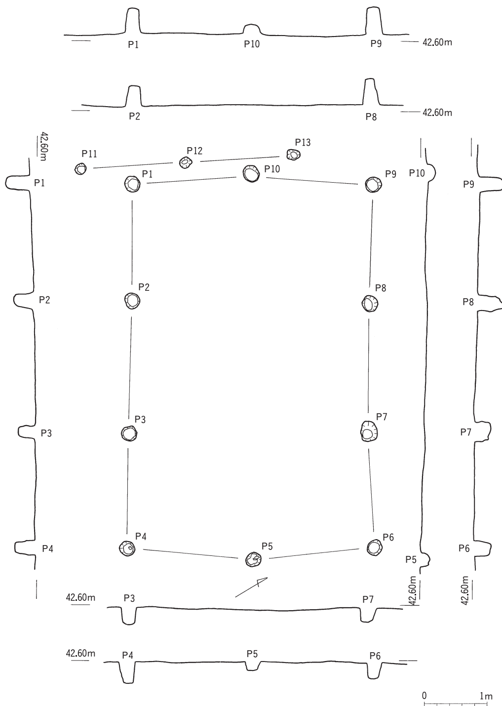
第50図 中世掘立柱建物跡（10）
