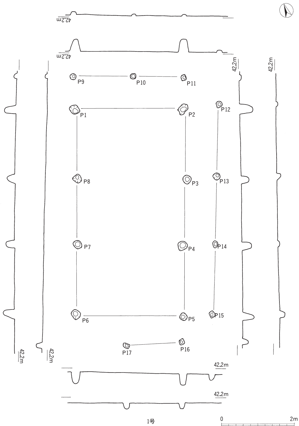
第16図 中世掘立柱建物跡（1）
