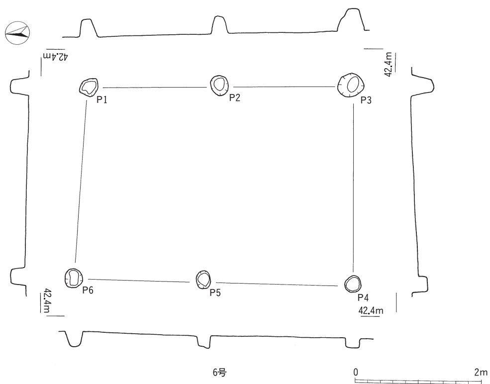
第20図 中世掘立柱建物跡（5）
