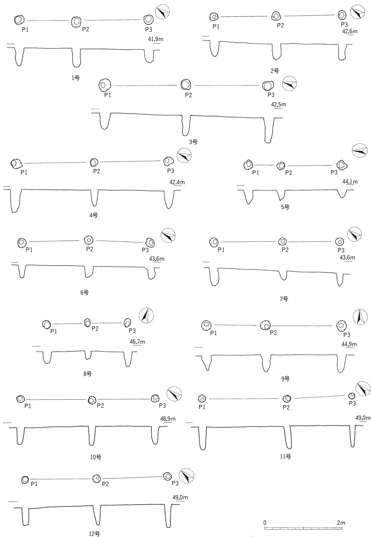
第14図 縄文時代晩期柱穴列 (1)
