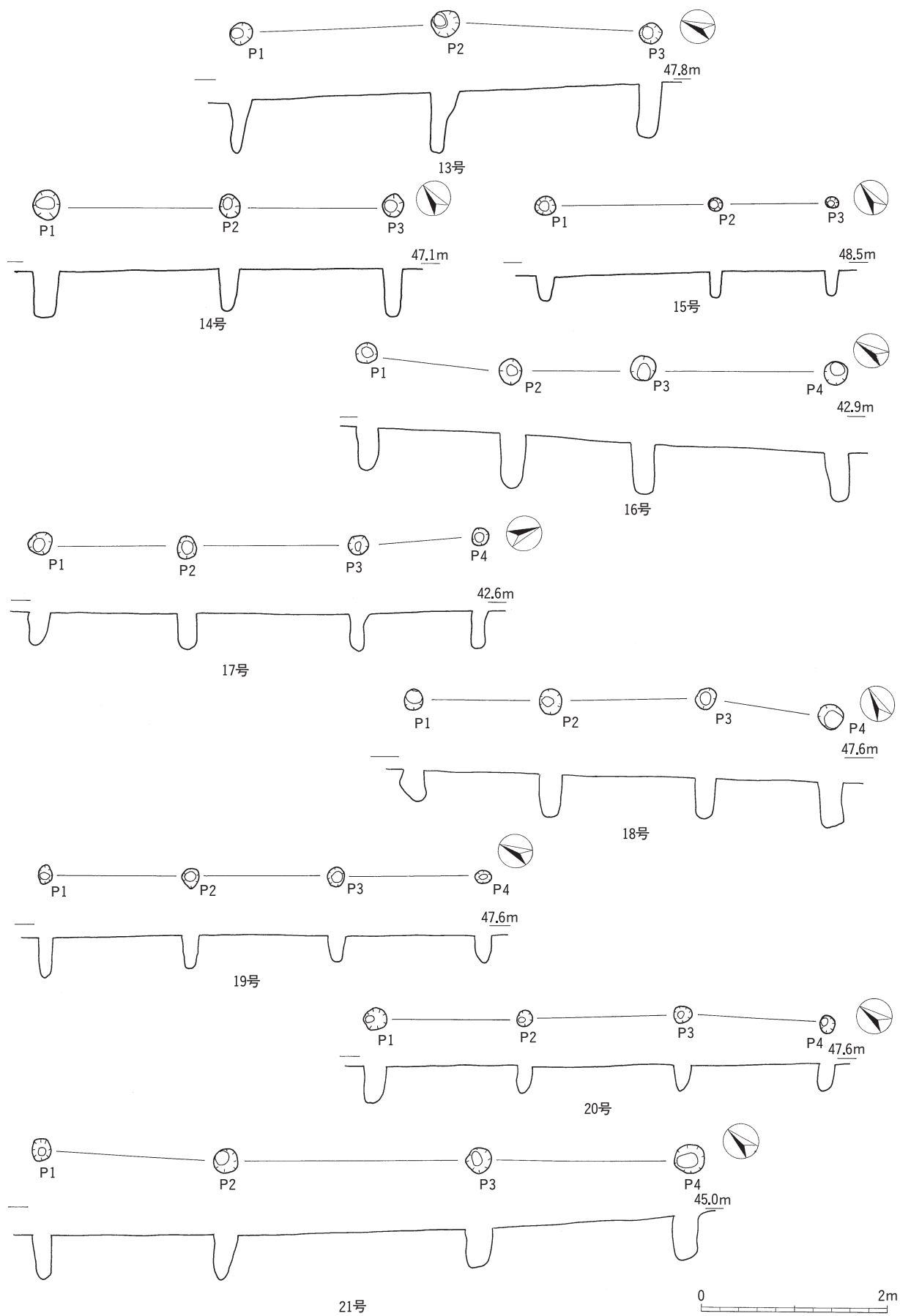
第15図 縄文時代晩期柱穴列（2）
