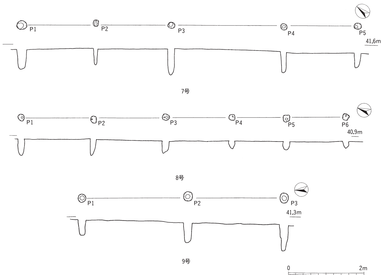
第10図 縄文時代晩期柱穴列（2）
