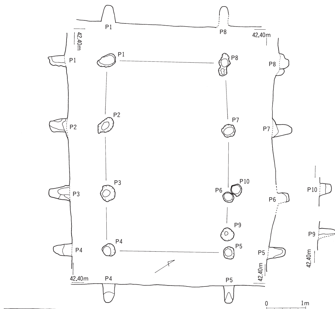
第51図 中世掘立柱建物跡 (11)
