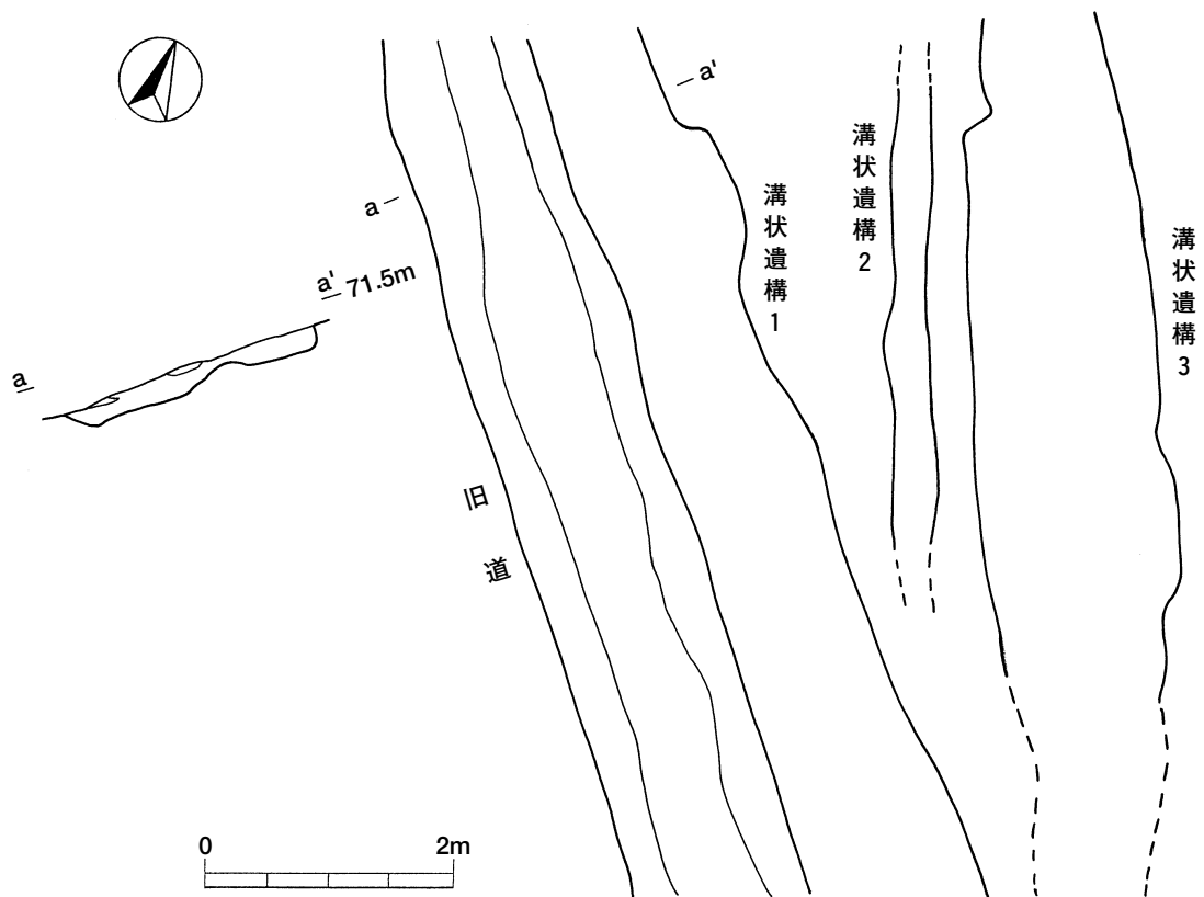
第61図 旧道・溝状遺構 1 ～ 3 実測図
