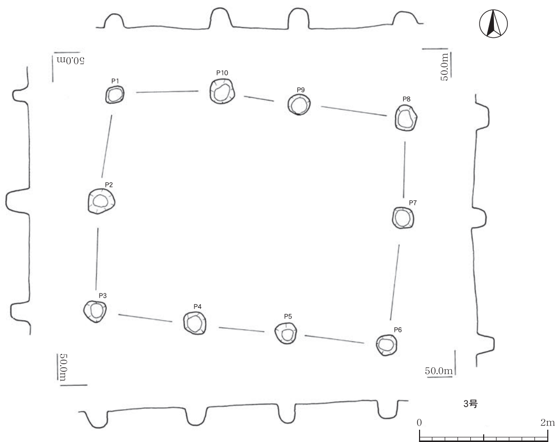
第137図 掘立柱建物跡 3号
