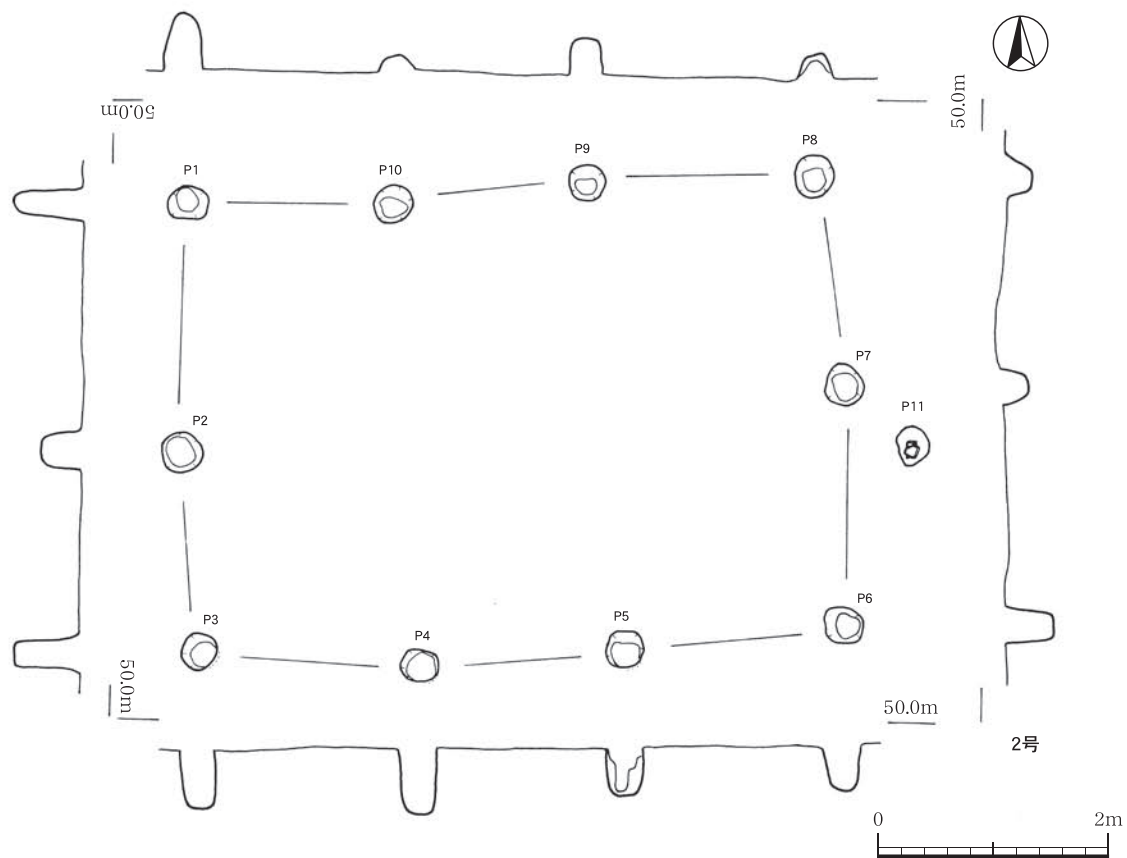
第136図 掘立柱建物跡 1・2号
