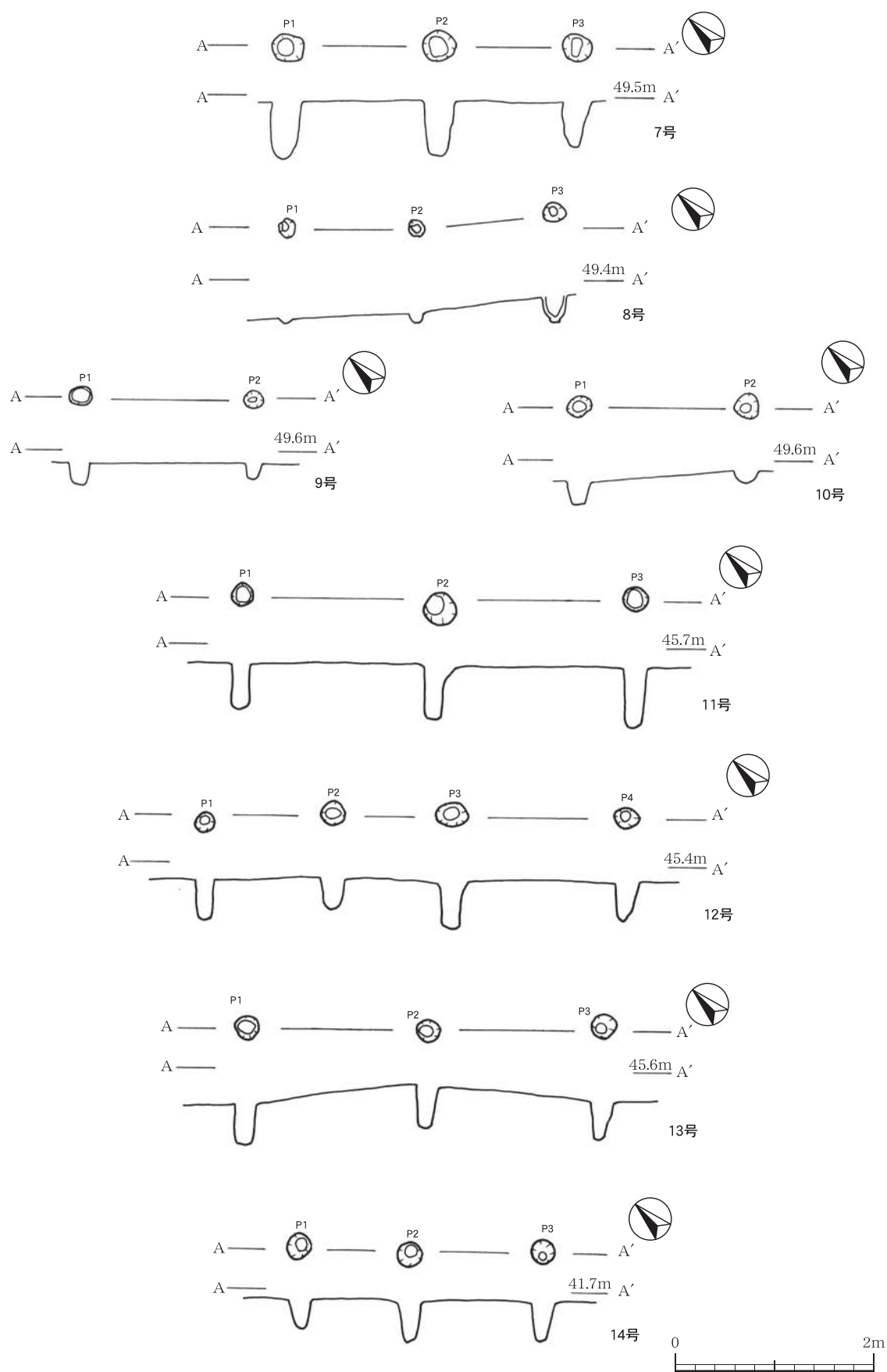
第95図 柱穴列 7 ~ 14 号
