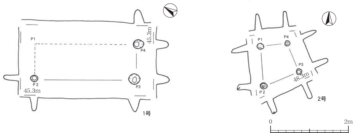
第93図 掘立柱建物跡 1・2号
