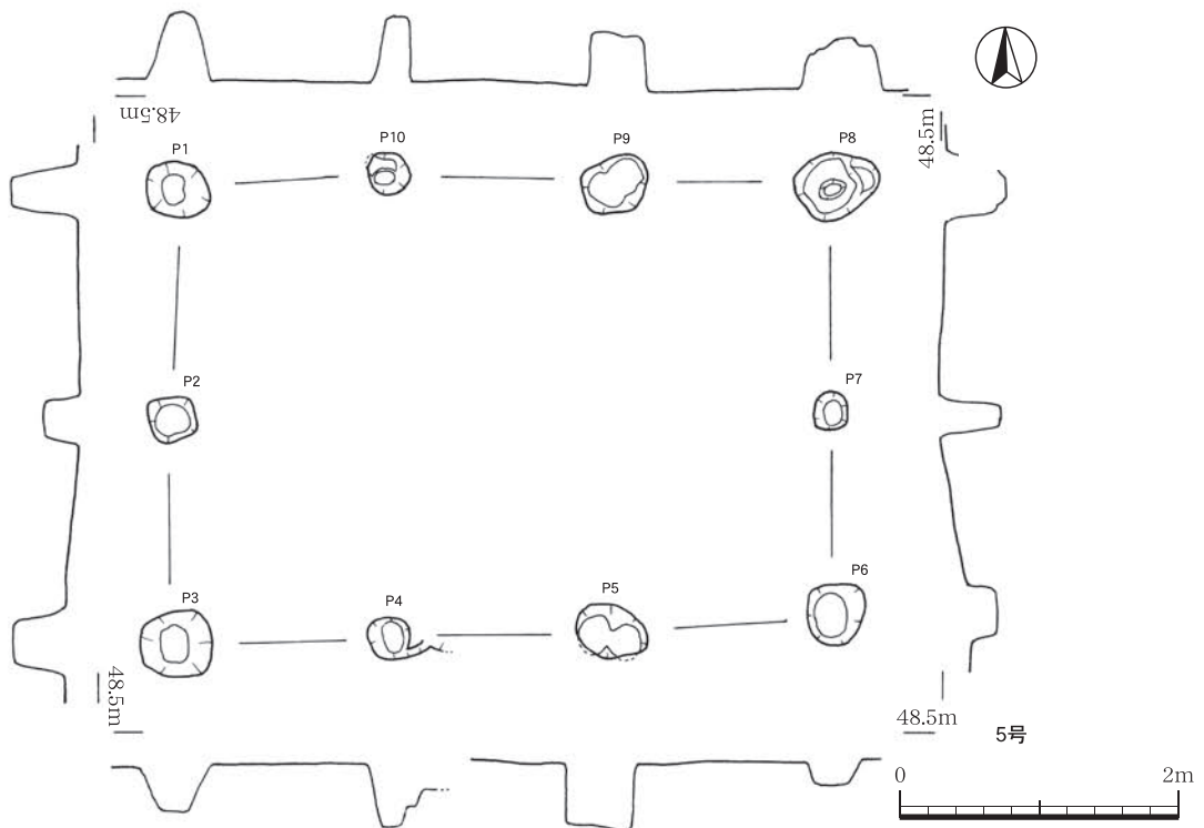
第138図 掘立柱建物跡 4・5号
