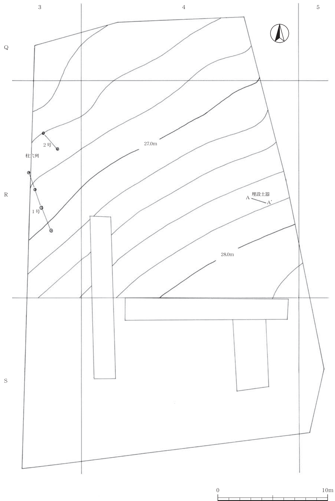
第14図 縄文時代晩期遺構配置図
