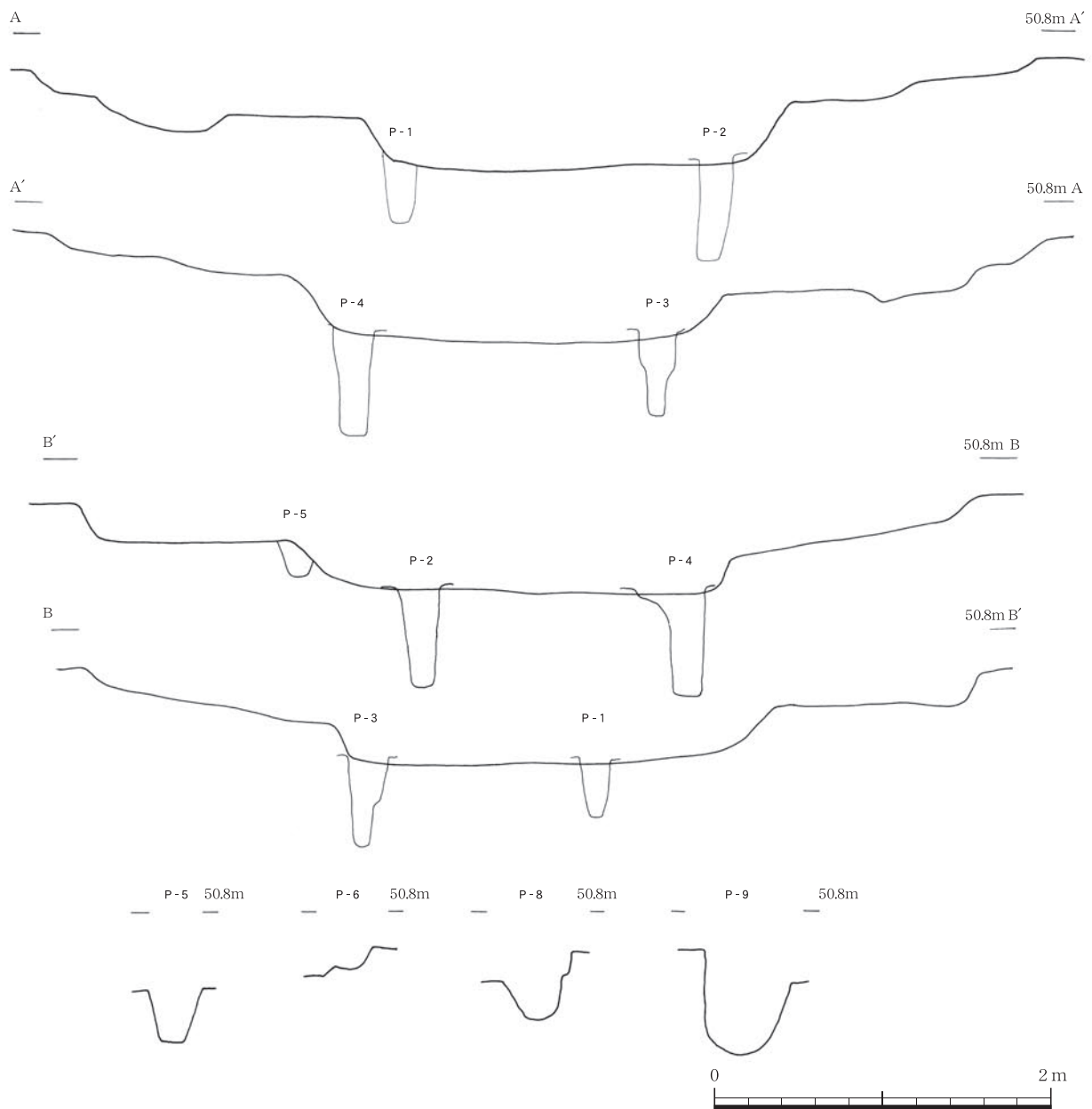
第105図 2号竪穴住居跡断面図
