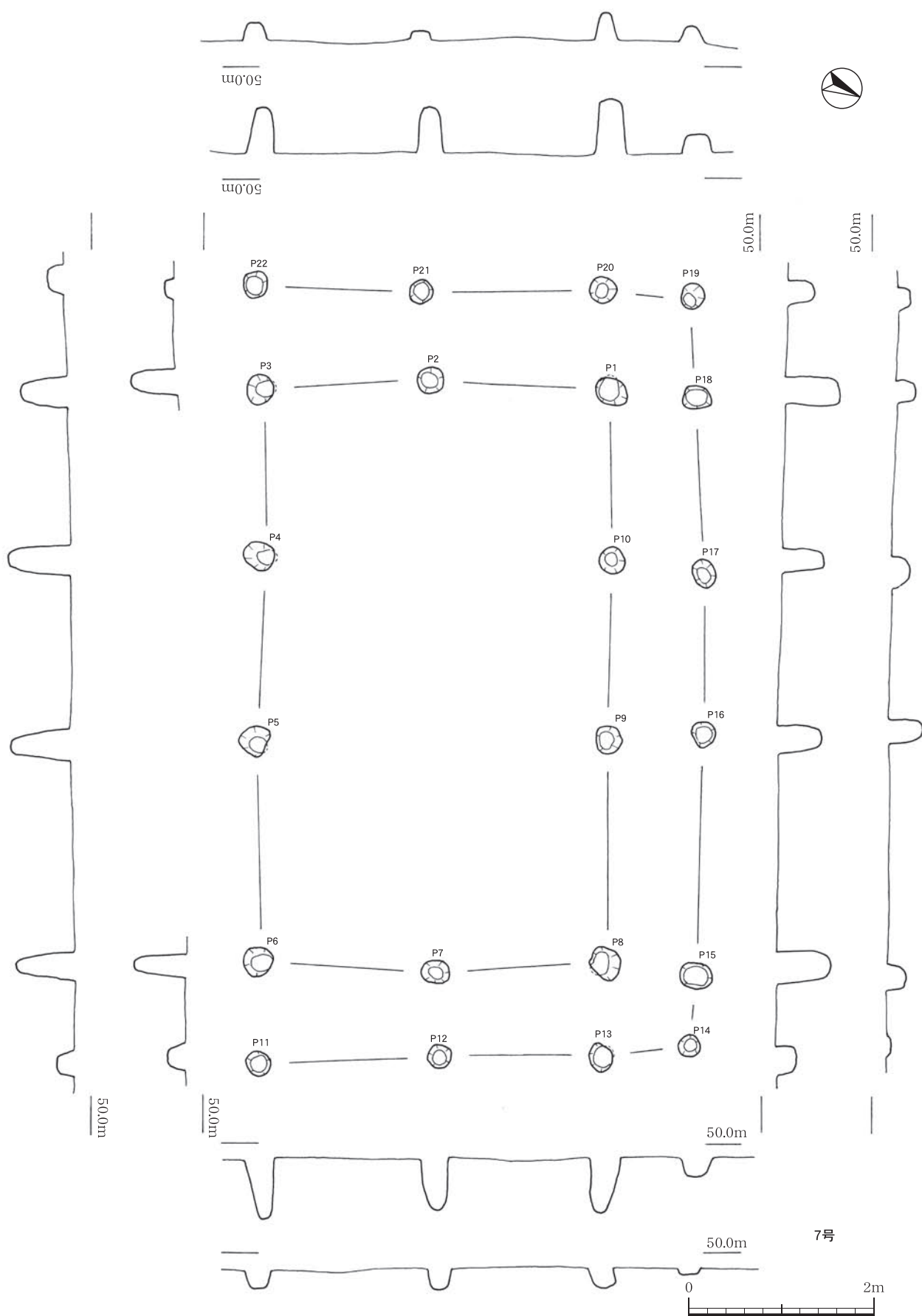
第140図 掘立柱建物跡 7号
