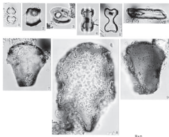
図版 1 植物珪酸体
