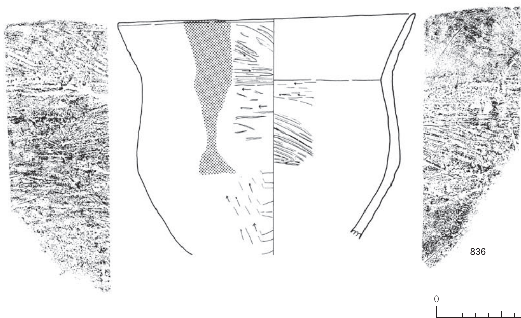
第89図 埋設土器 1号・2号実測図
