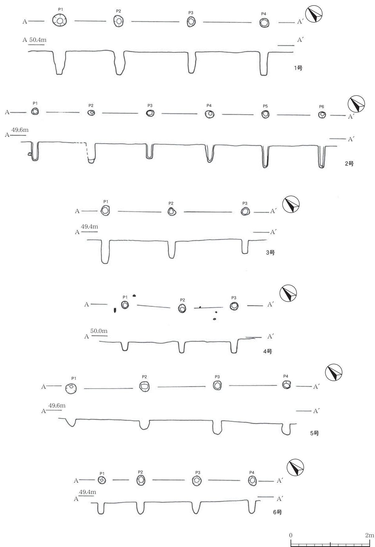
第94図 柱穴列 1～6号
