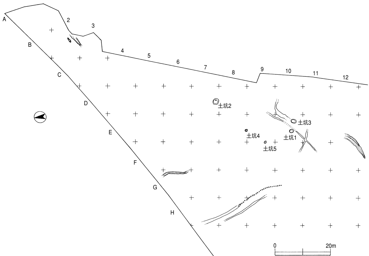
第75図 原村Ⅰ遺跡遺構配置図
