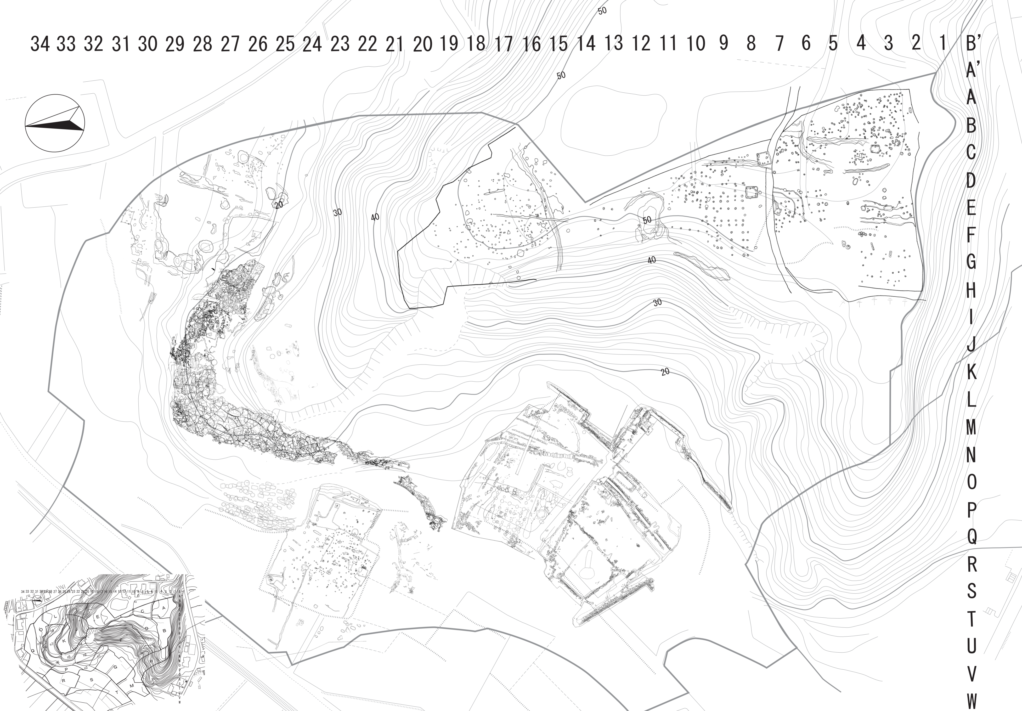
柁城跡遺構配置図
