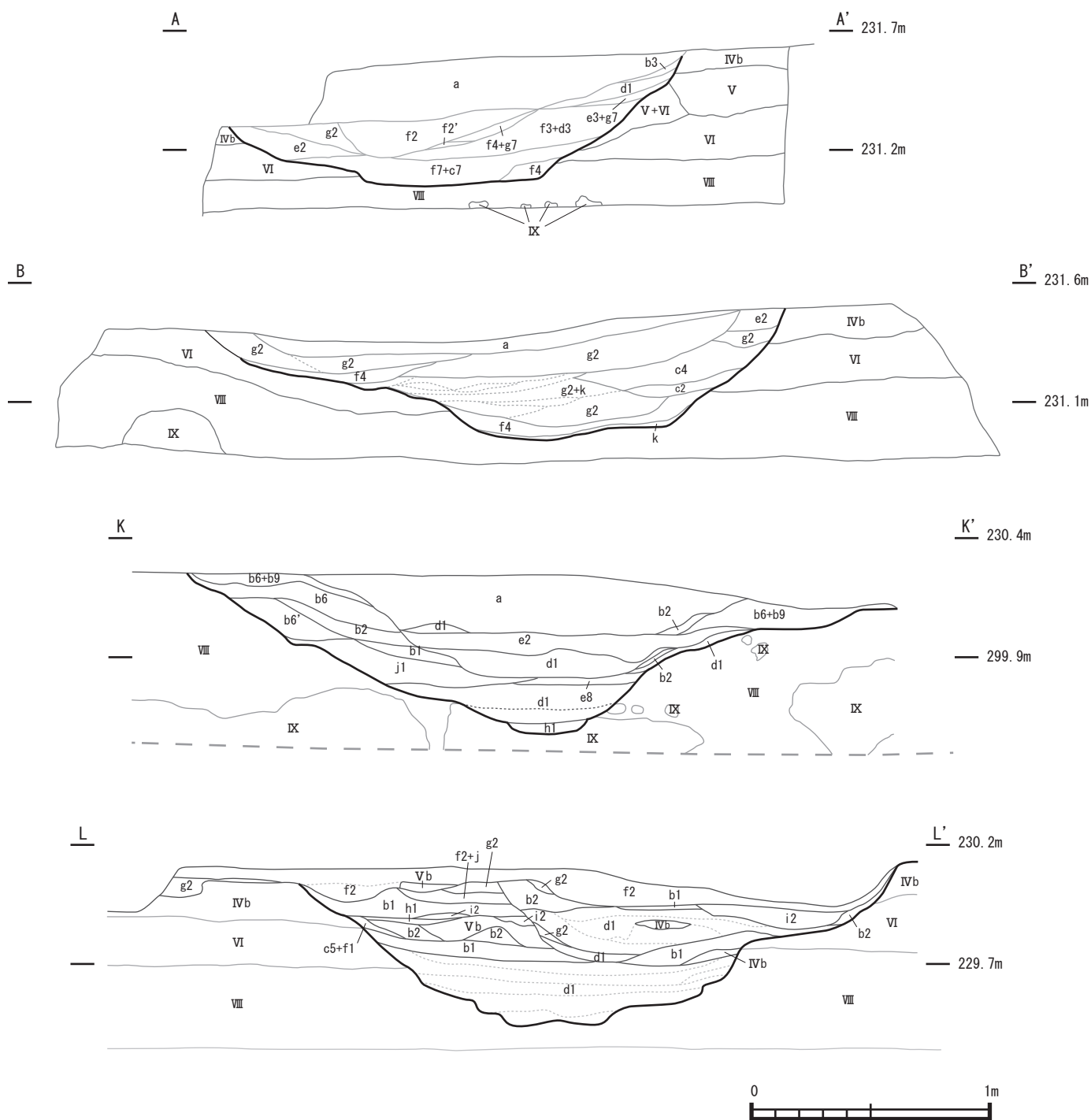
第112図 近世以降の道跡断面図
