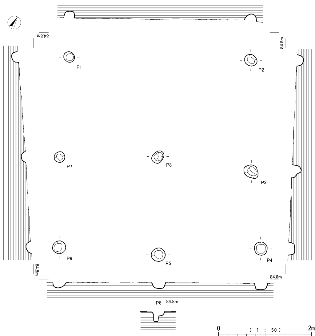
第229図 掘立柱建物跡5号
