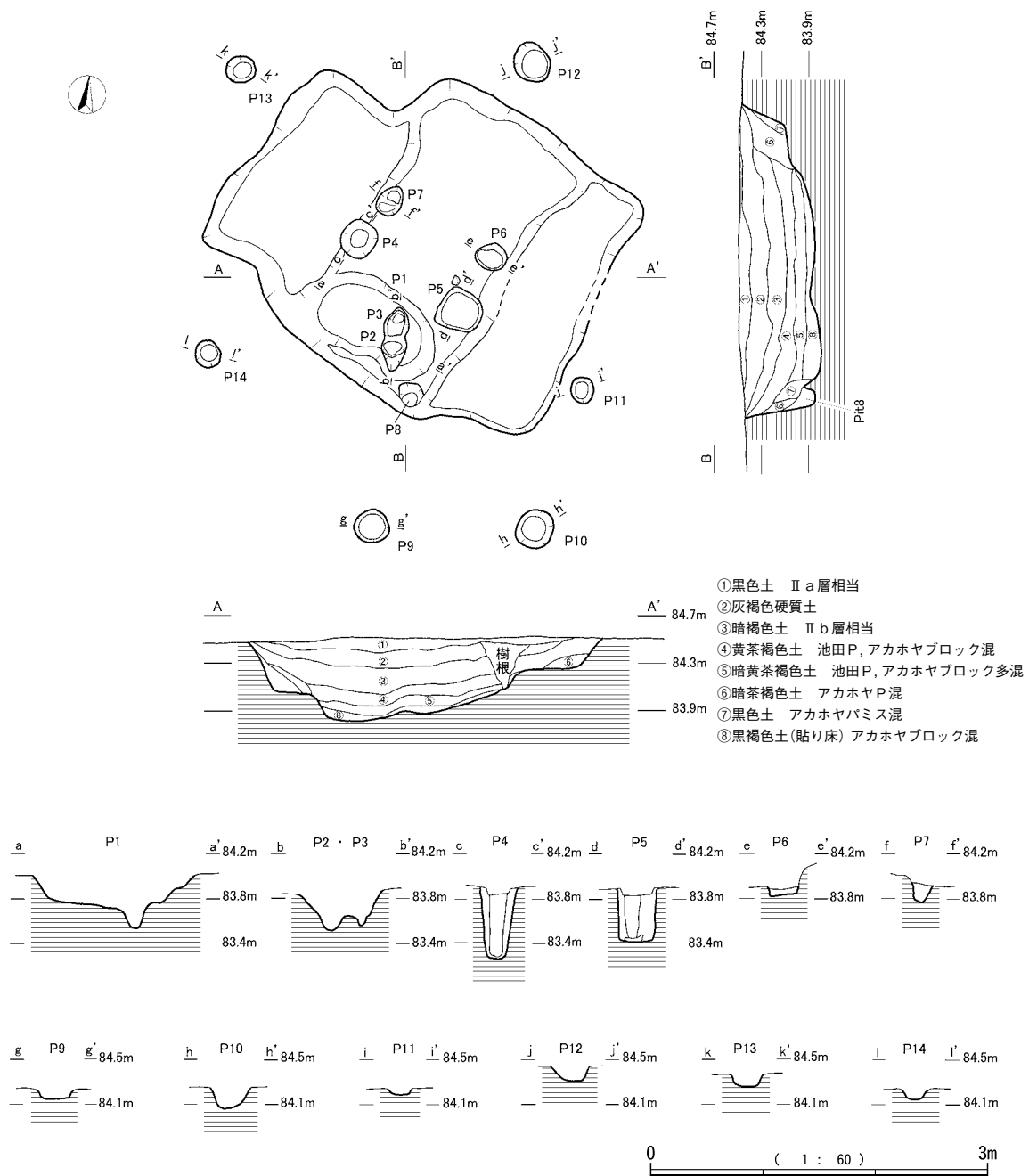
第201図 竪穴住居跡3号
