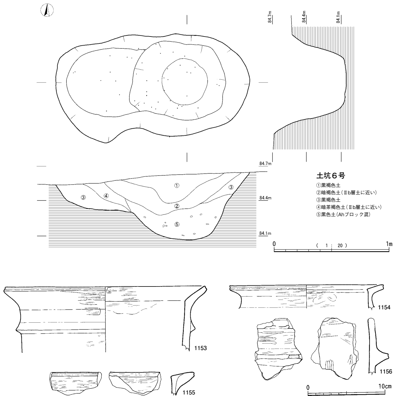
第235図 土坑6号及び出土遺物
