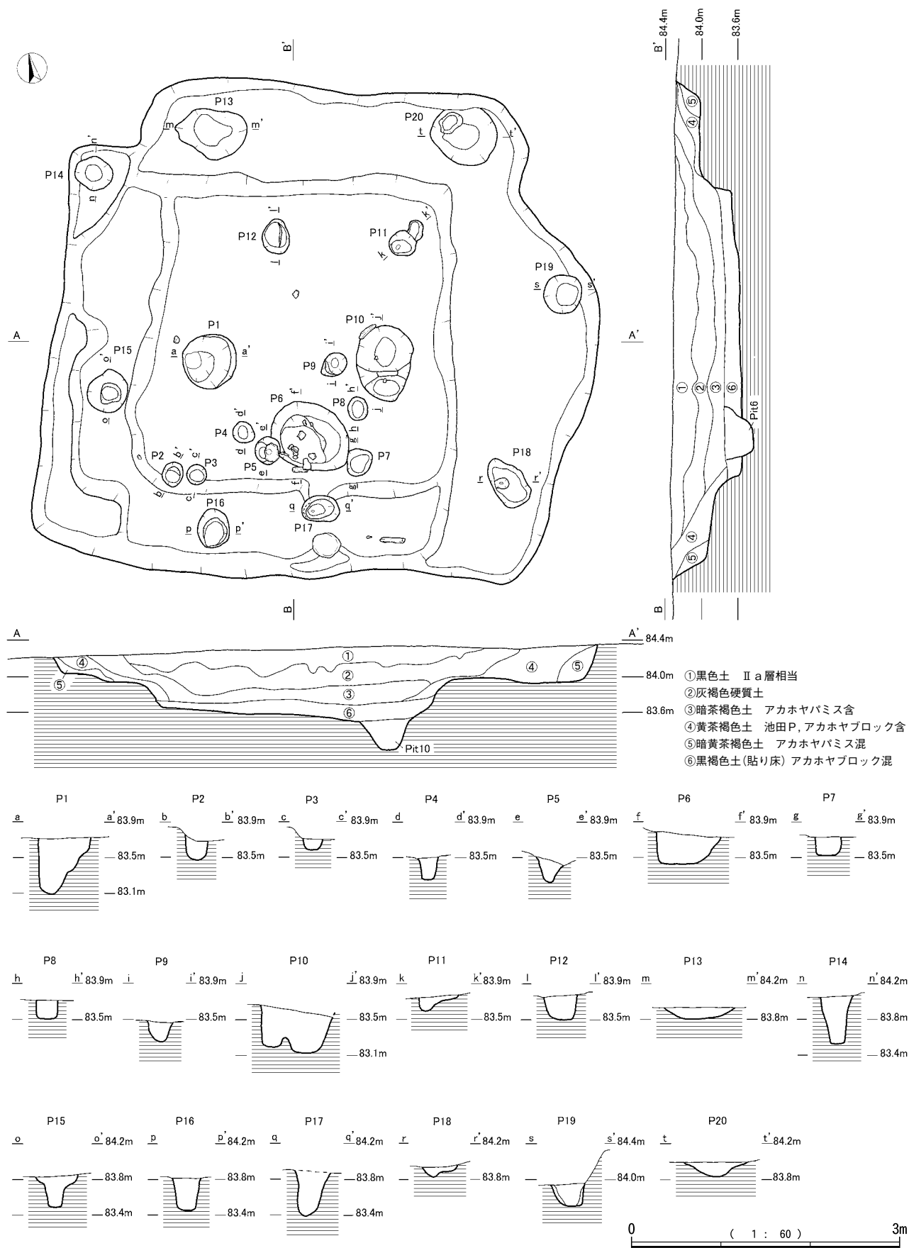
第193図 竪穴住居跡2号
