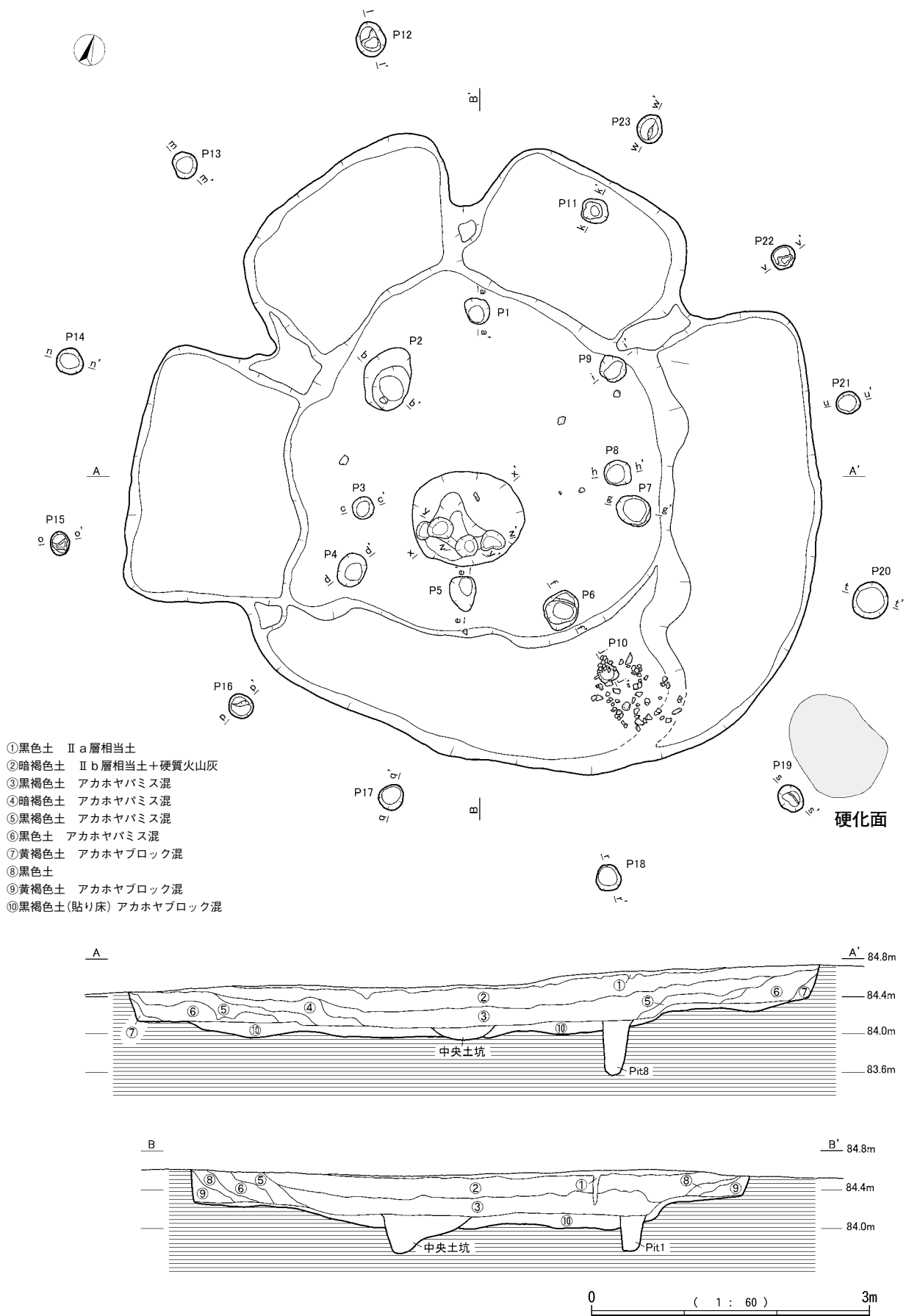
第187図 竪穴住居跡1号(1)
