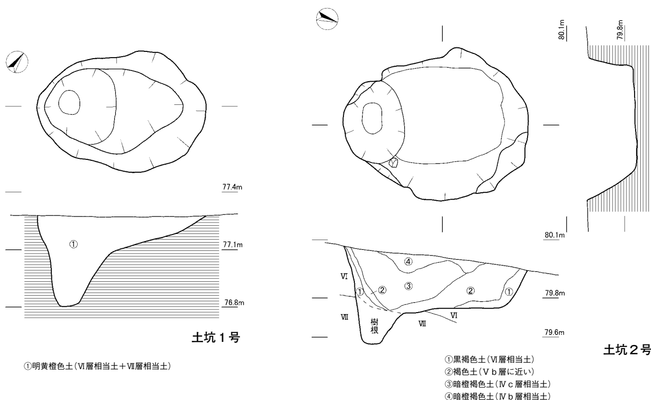
第96図 土坑 1・2号
