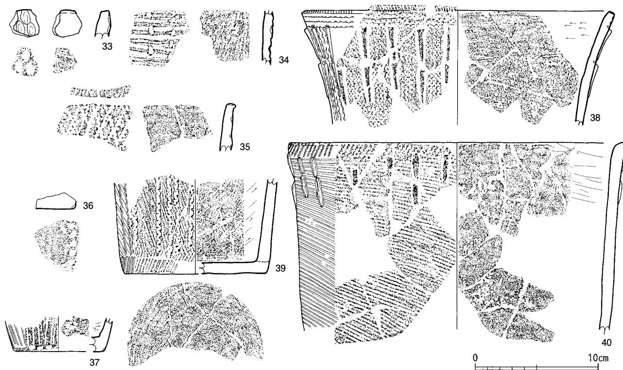
第100図 縄文時代早期の土器 (1)
