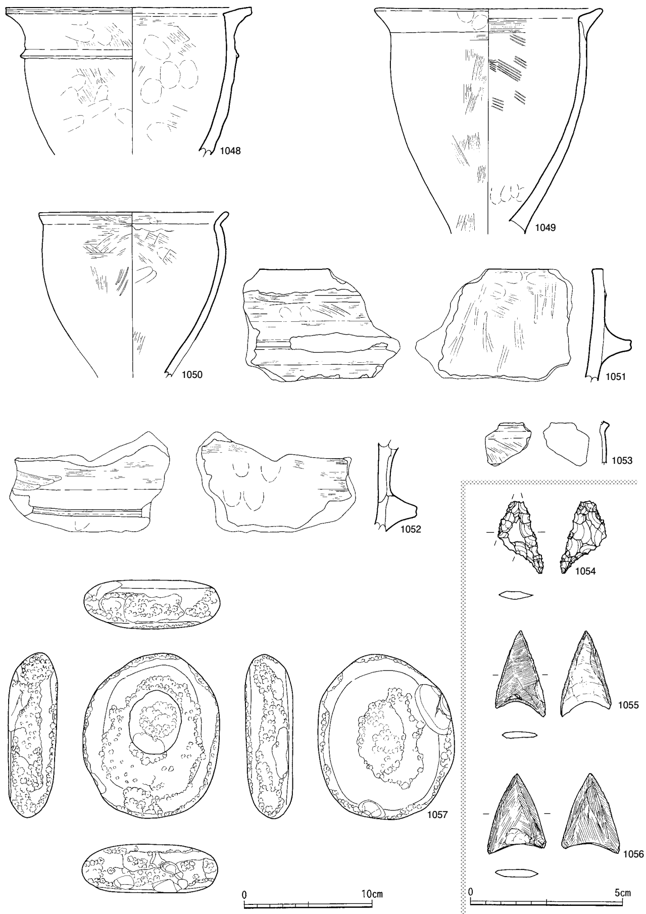
第209图 竖穴住居跡4号出土遺物(3)
