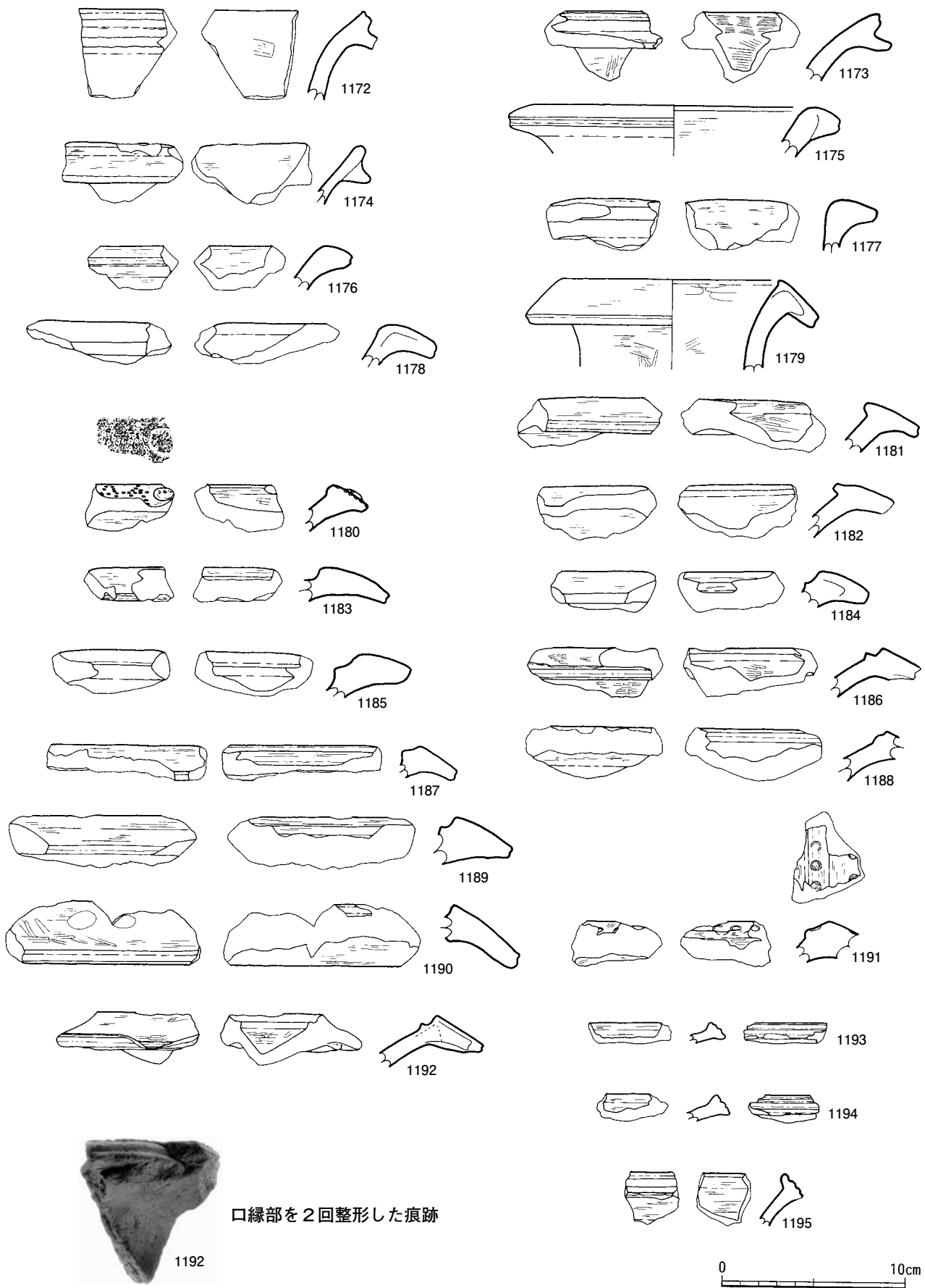
第241図 弥生時代中期の土器（2）
