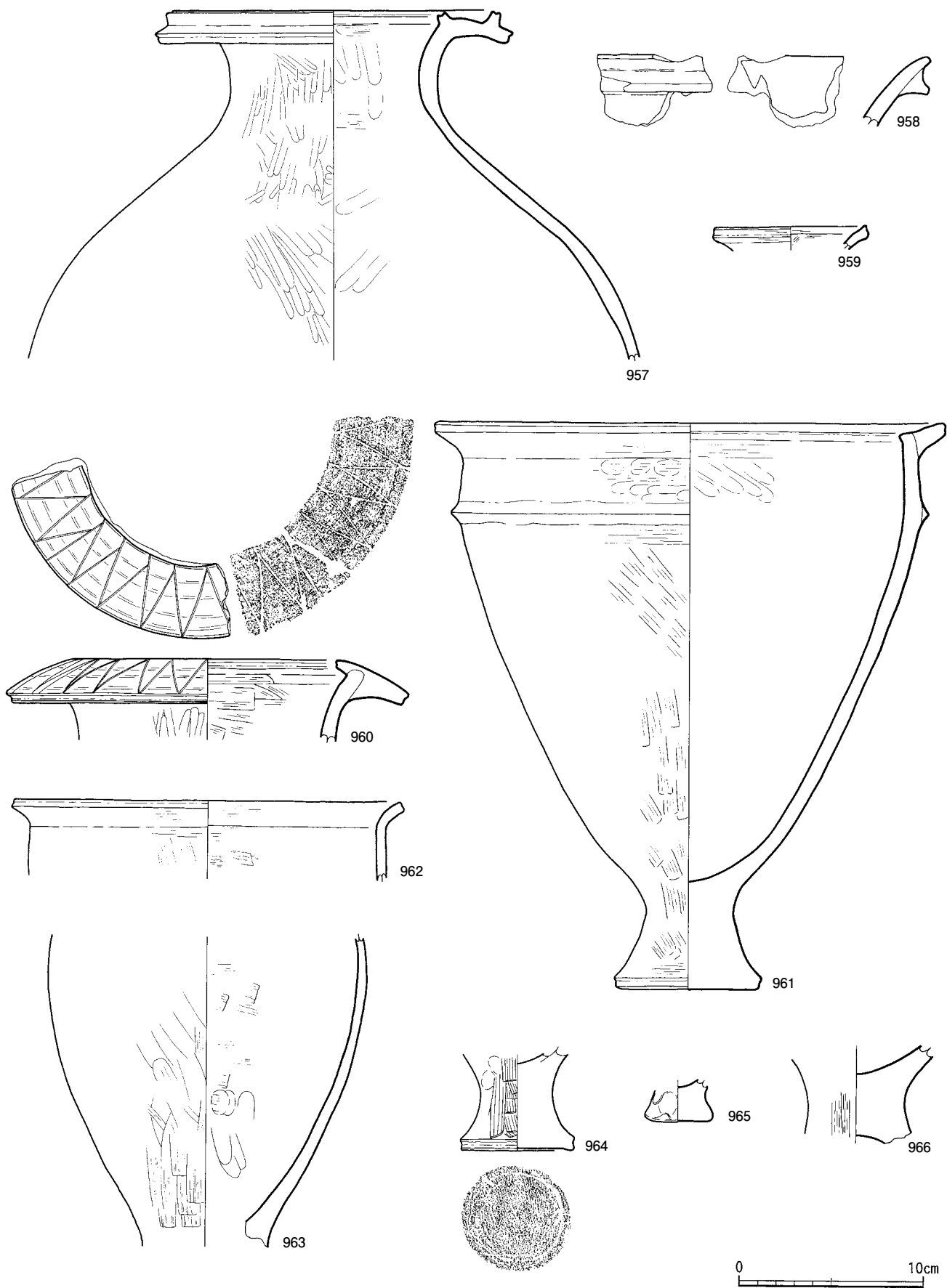
第190図 竪穴住居跡1号出土遺物(1)
