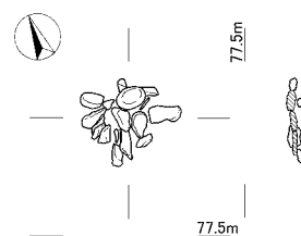
集石41号
