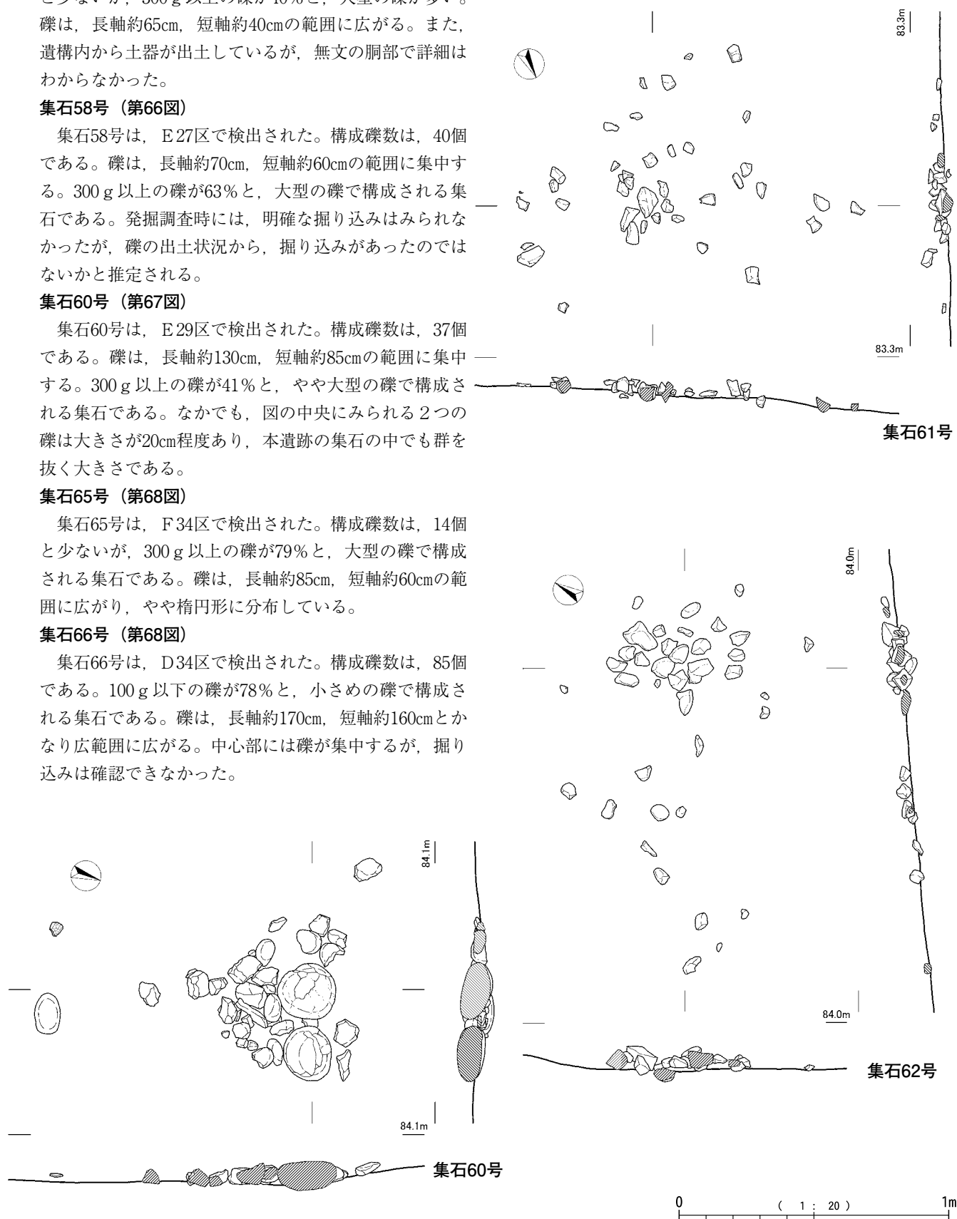
第67図 集石60～62号
