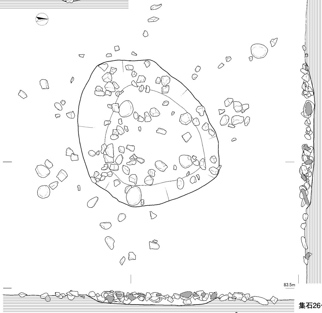
第54図 集石24～26号
