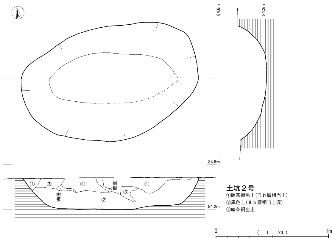
第232図 土坑 2 号
