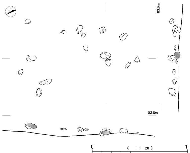
第34図 礫群
