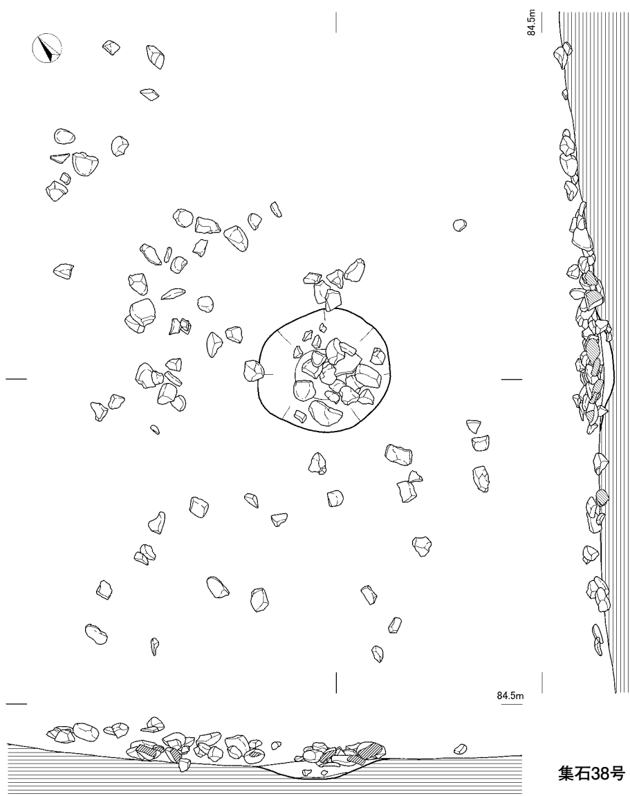
第59図 集石36 ~ 38号
