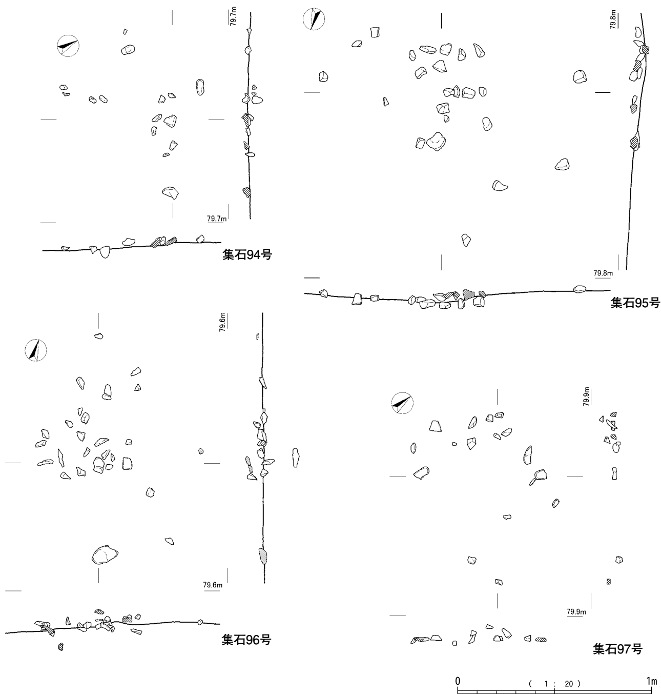
第76図 集石94～97号
