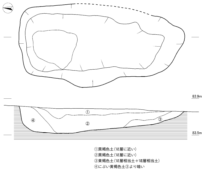
土坑5号
