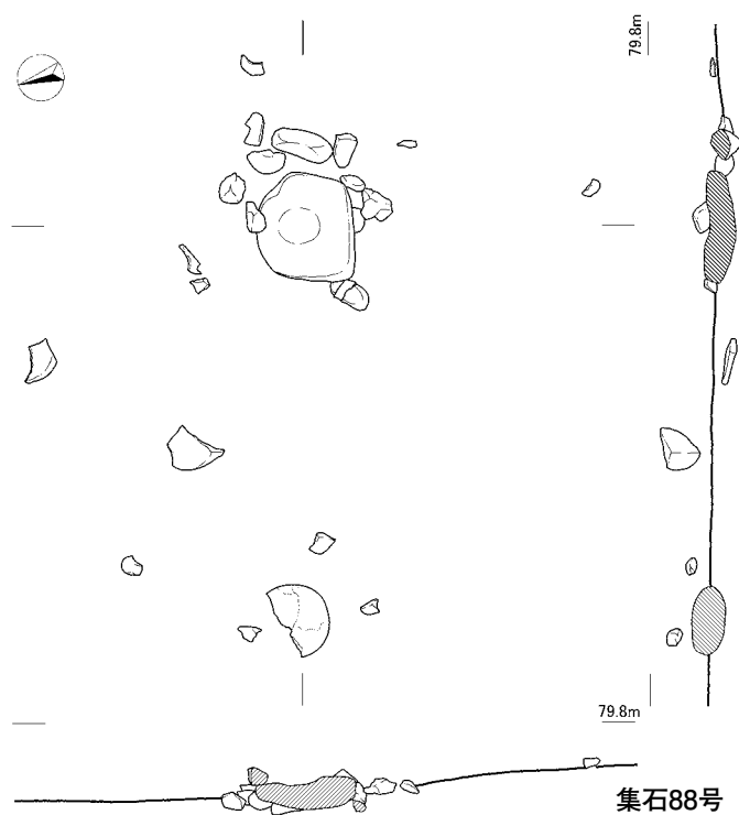
第73図 集石84 ~ 88号
