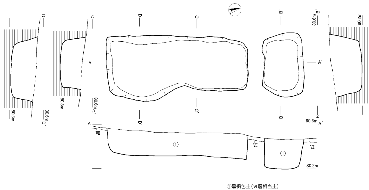
土坑3・4号
