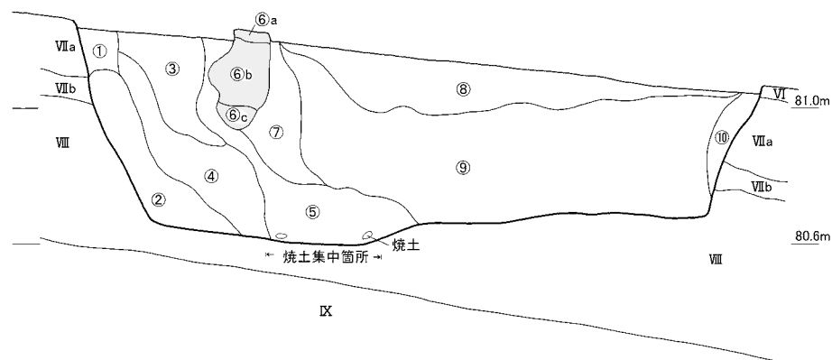
連穴土坑2号
