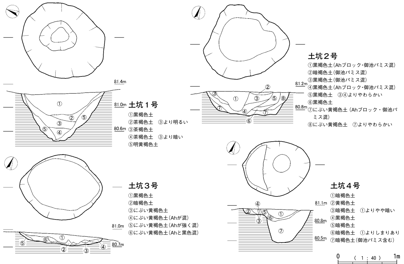
第182図 土坑1～4号
