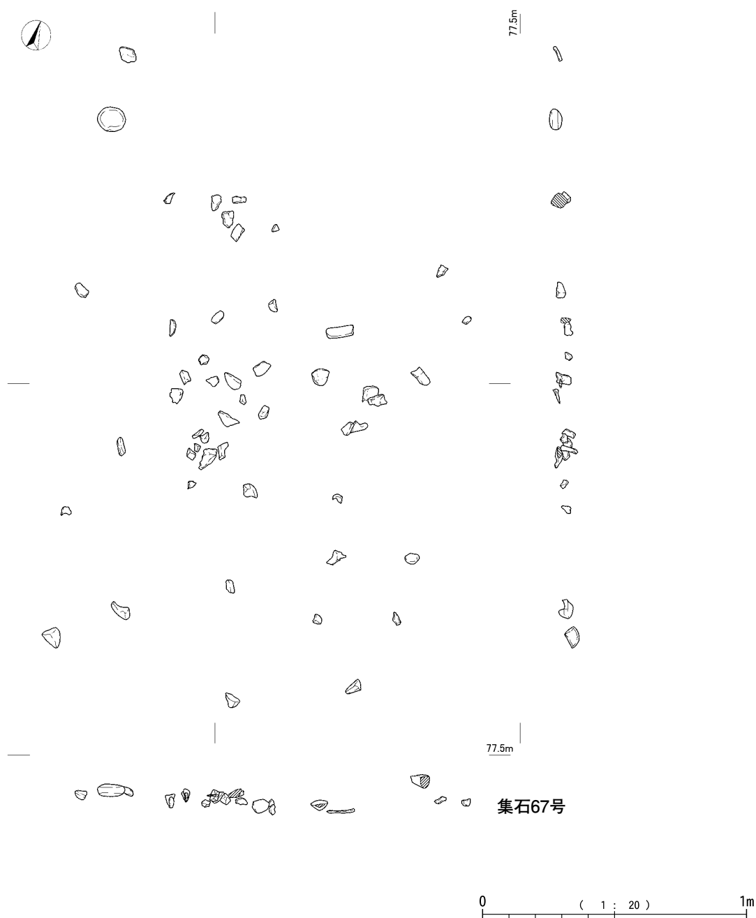
第69図 集石67号
