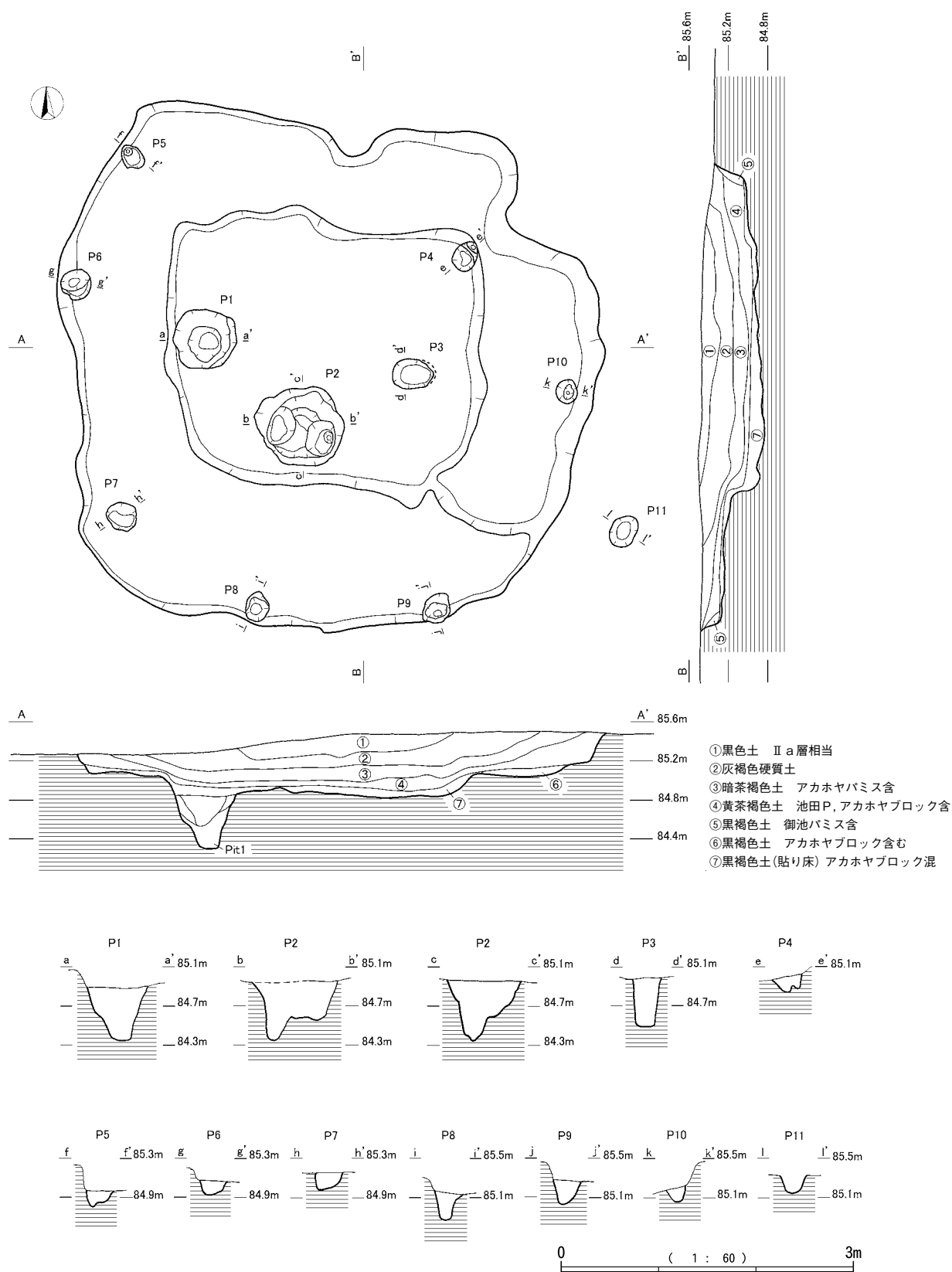
第211図 竪穴住居跡5号
