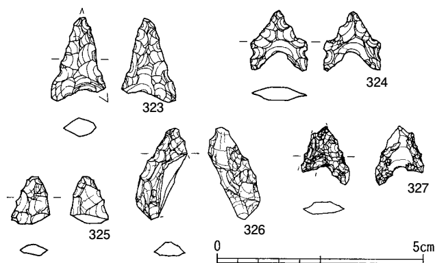
第126-2図 6ブロックの石器
