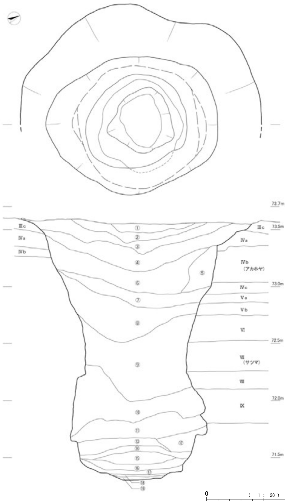
第16図 船迫遺跡 落し穴状遺構2号
