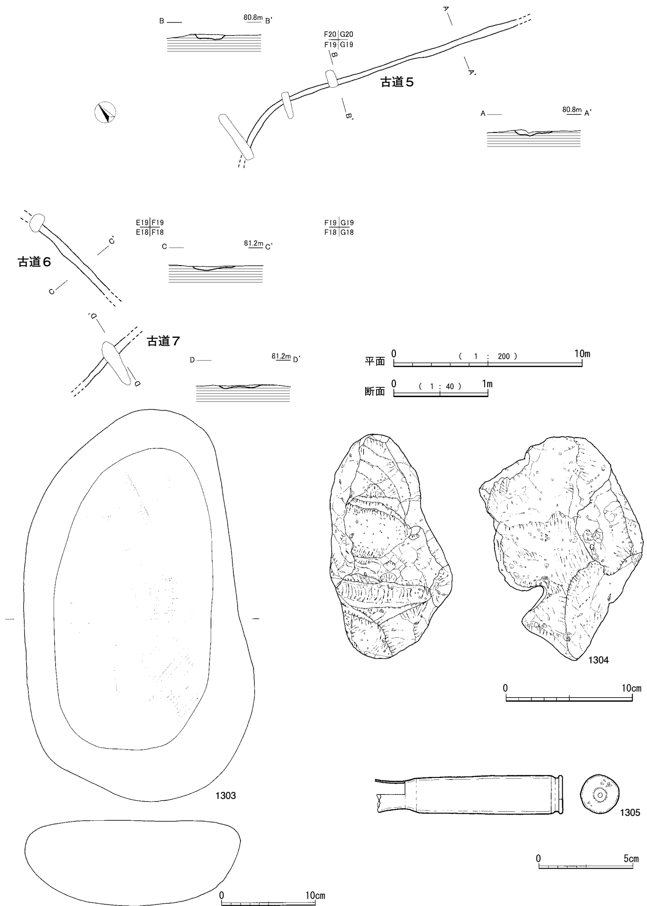
第258図 その他の遺構（6）及び出土遺物
