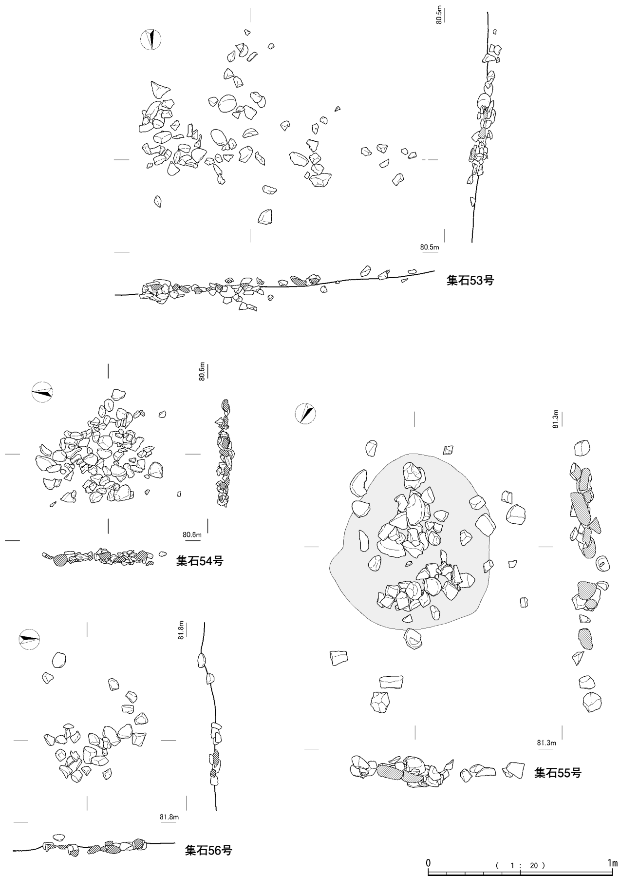
第65図 集石53 ~ 56号
