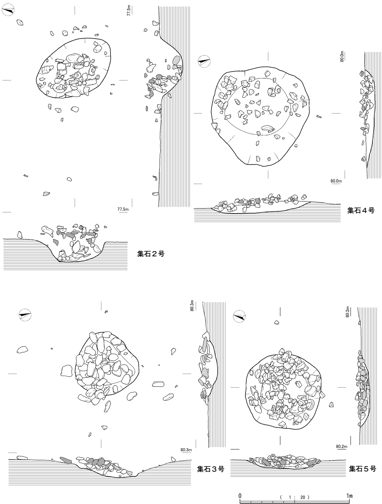
第47図 集石2～5号
