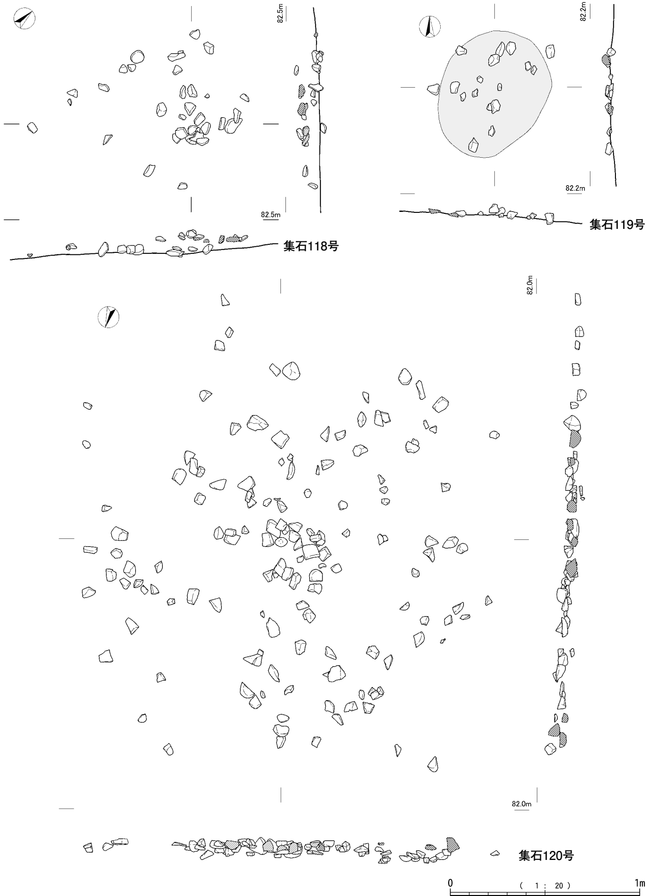
第83図 集石118 ~ 120号
