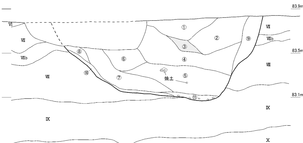
連穴土坑3号
