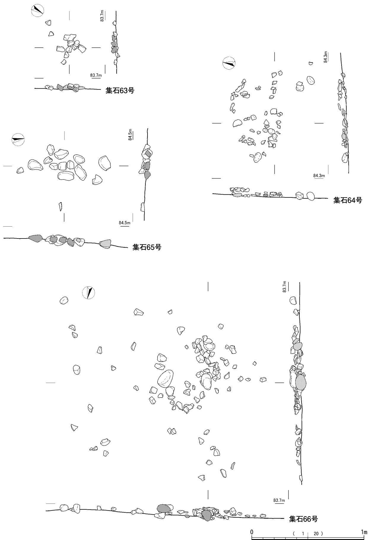
第68図 集石63 ~ 66号
