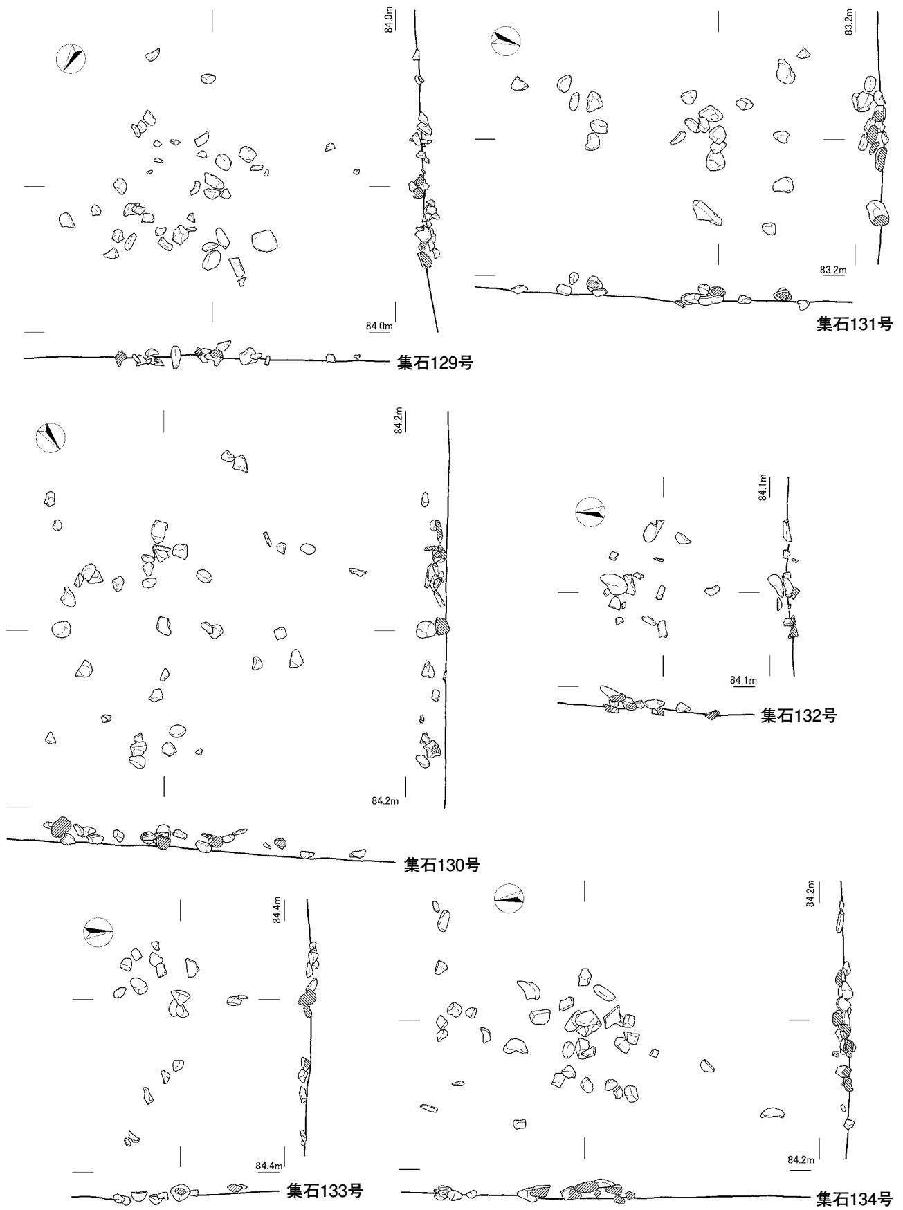
第86図 集石129 ~ 134号
