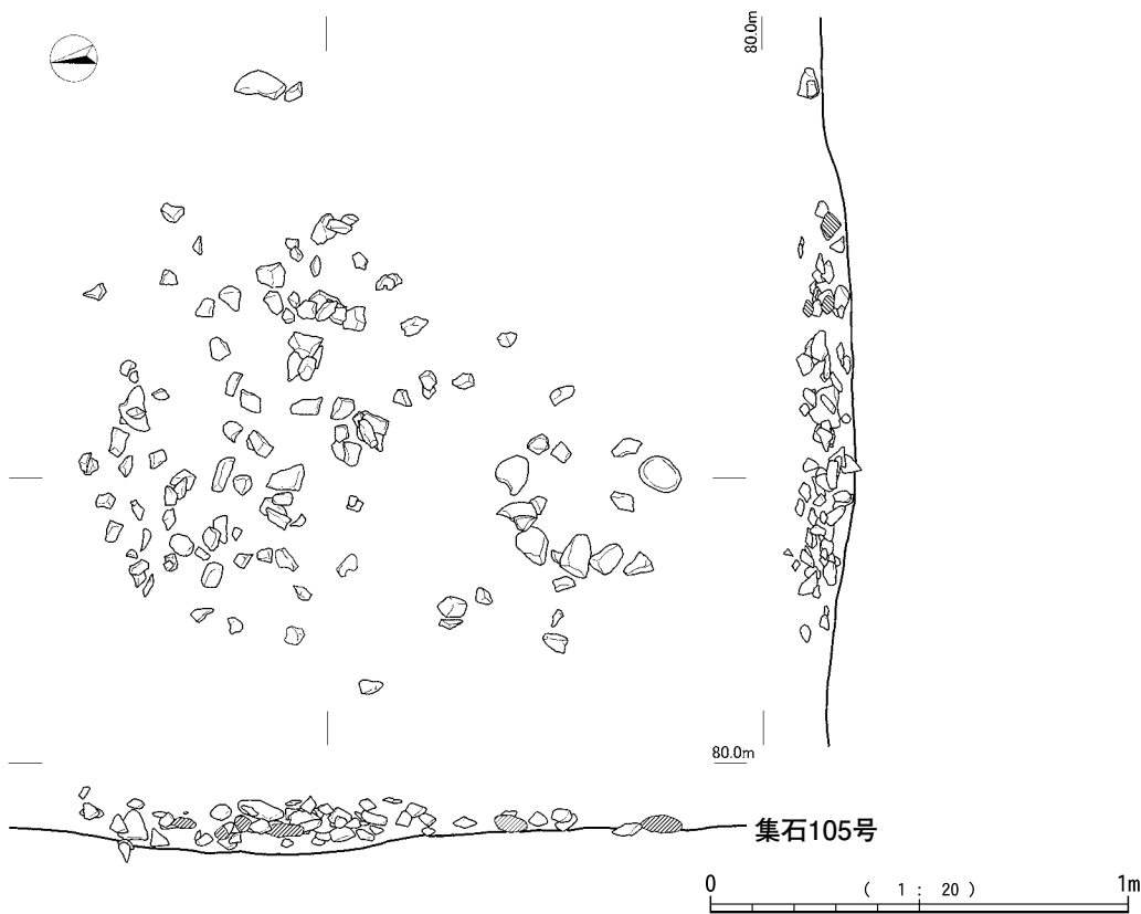
第78図 集石102 ~ 105号
