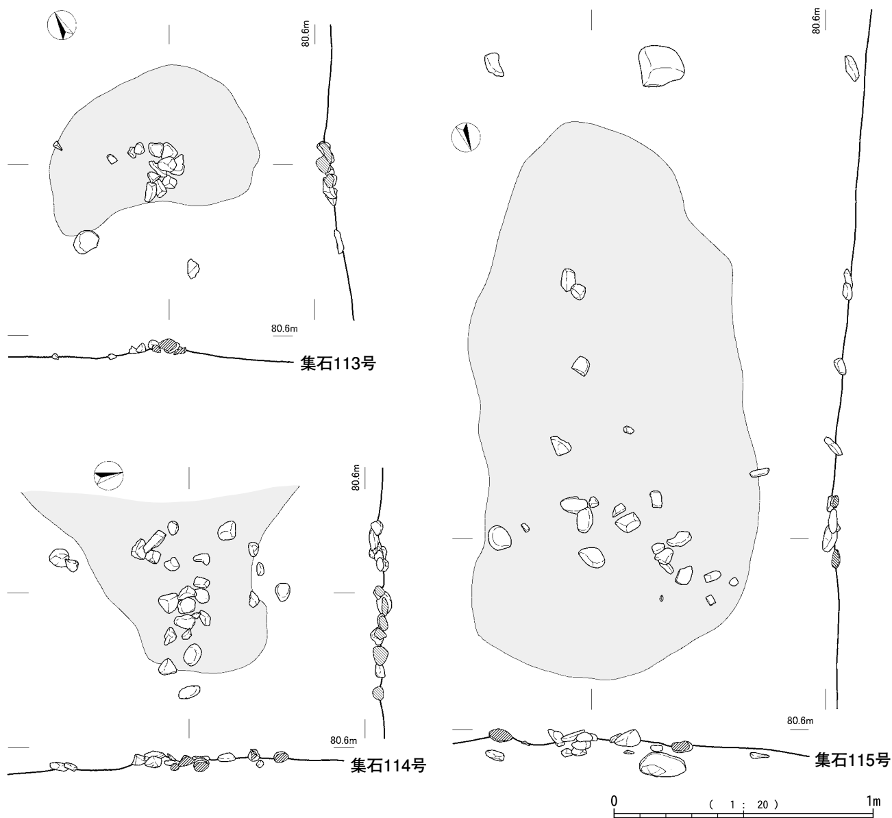
第81図 集石113～115号
