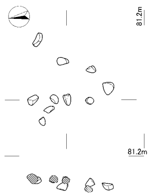
集石109号
