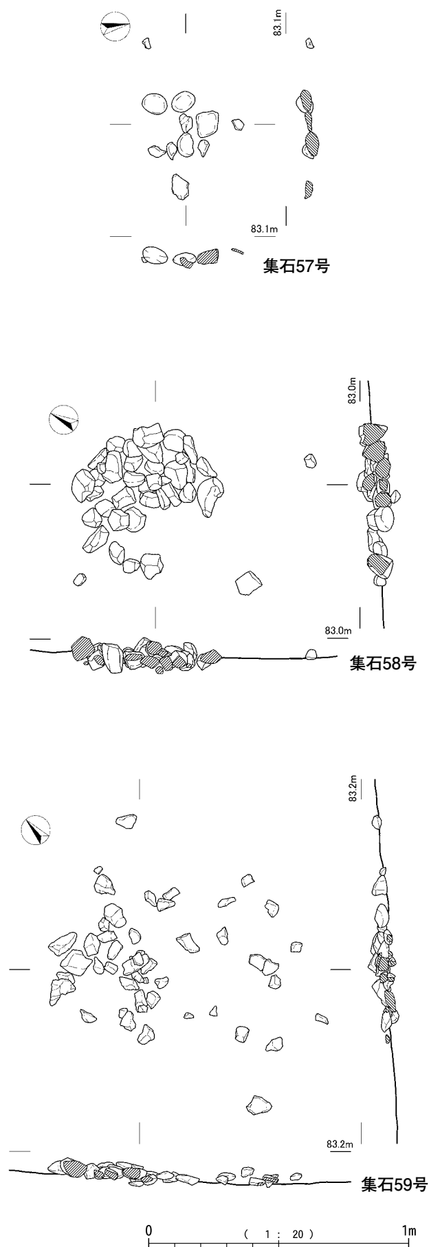
第66図 集石57～59号
