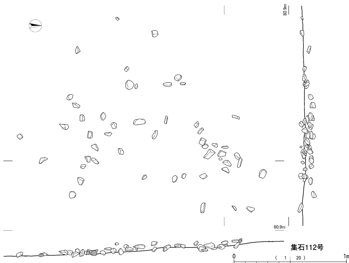
第80図 集石109 ~ 112号
