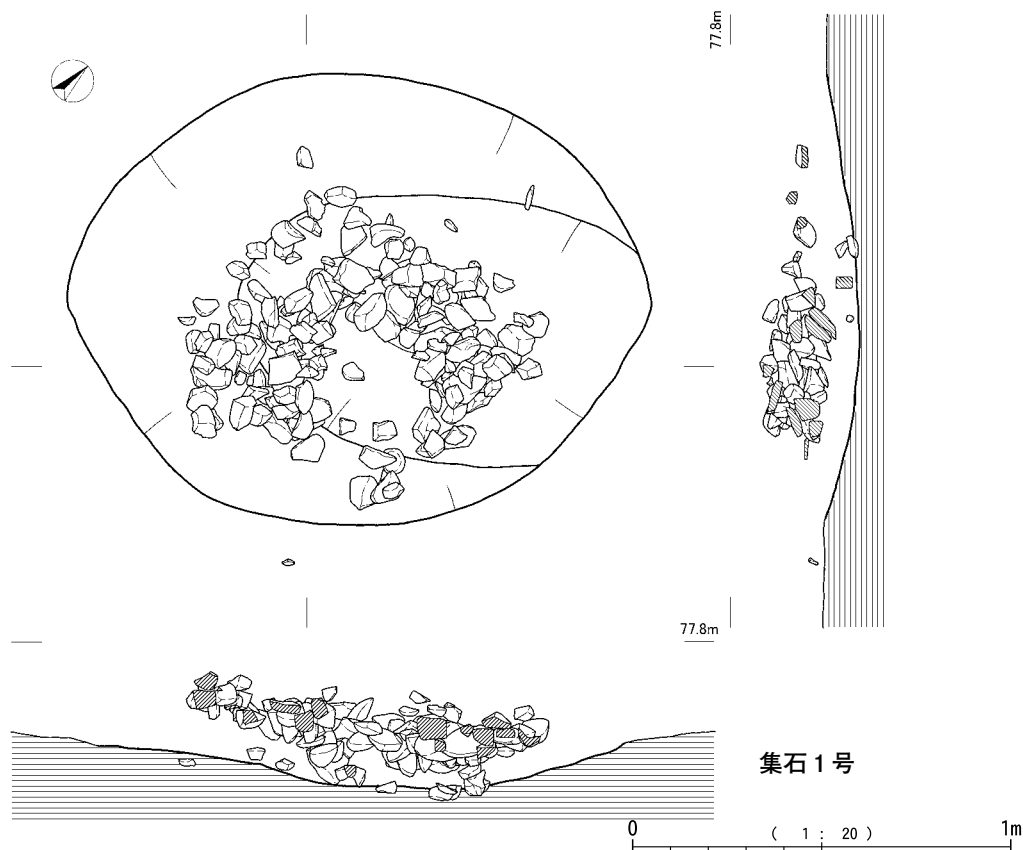
第46図 集石 1 号
