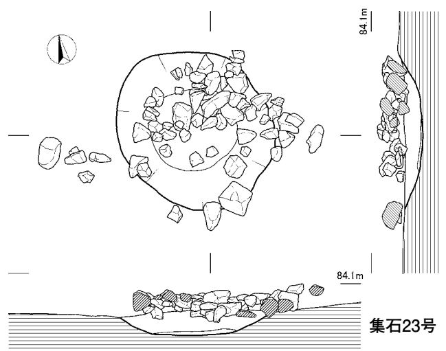
第53図 集石20～23号
