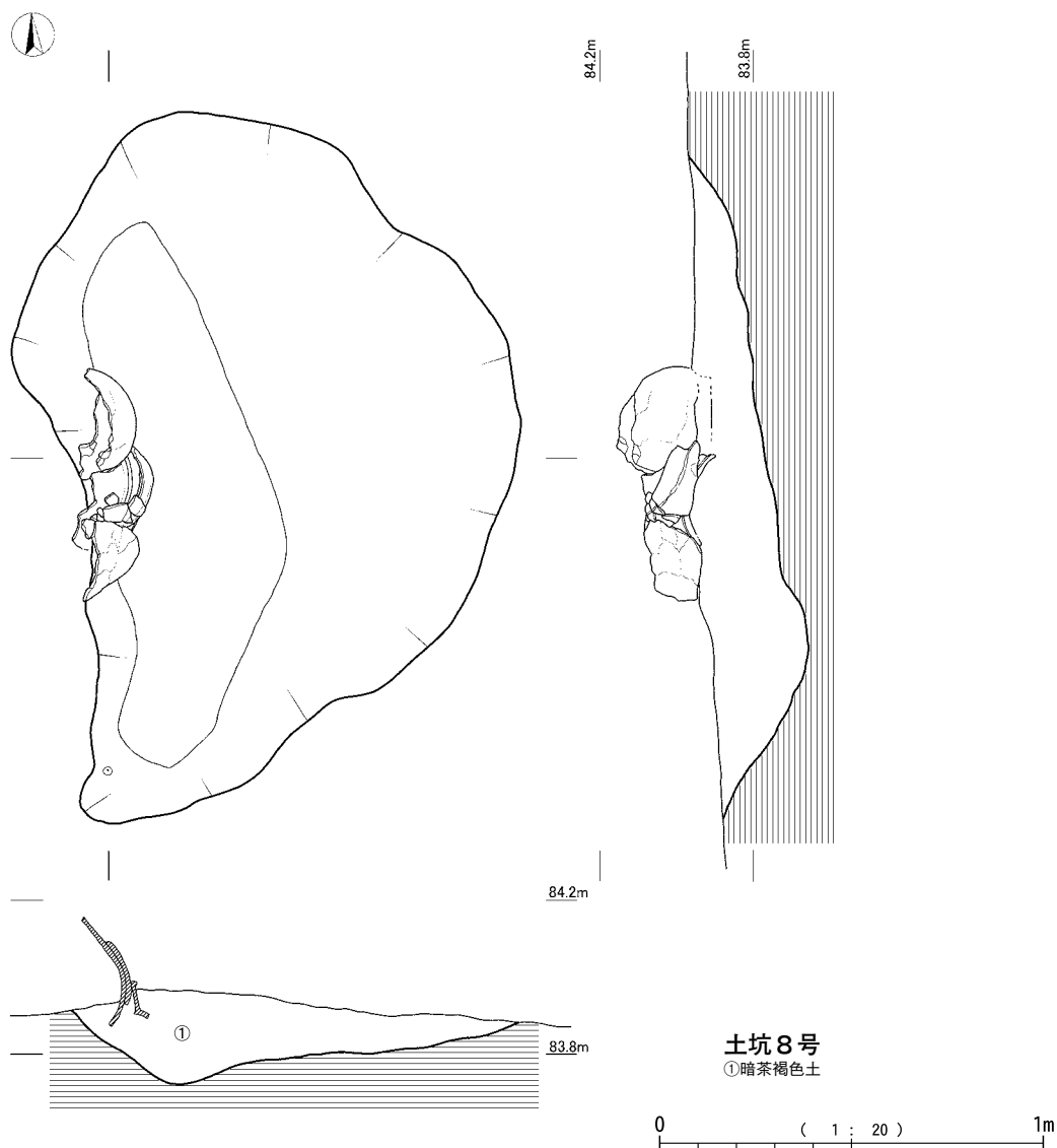
第238図 土坑 8号
