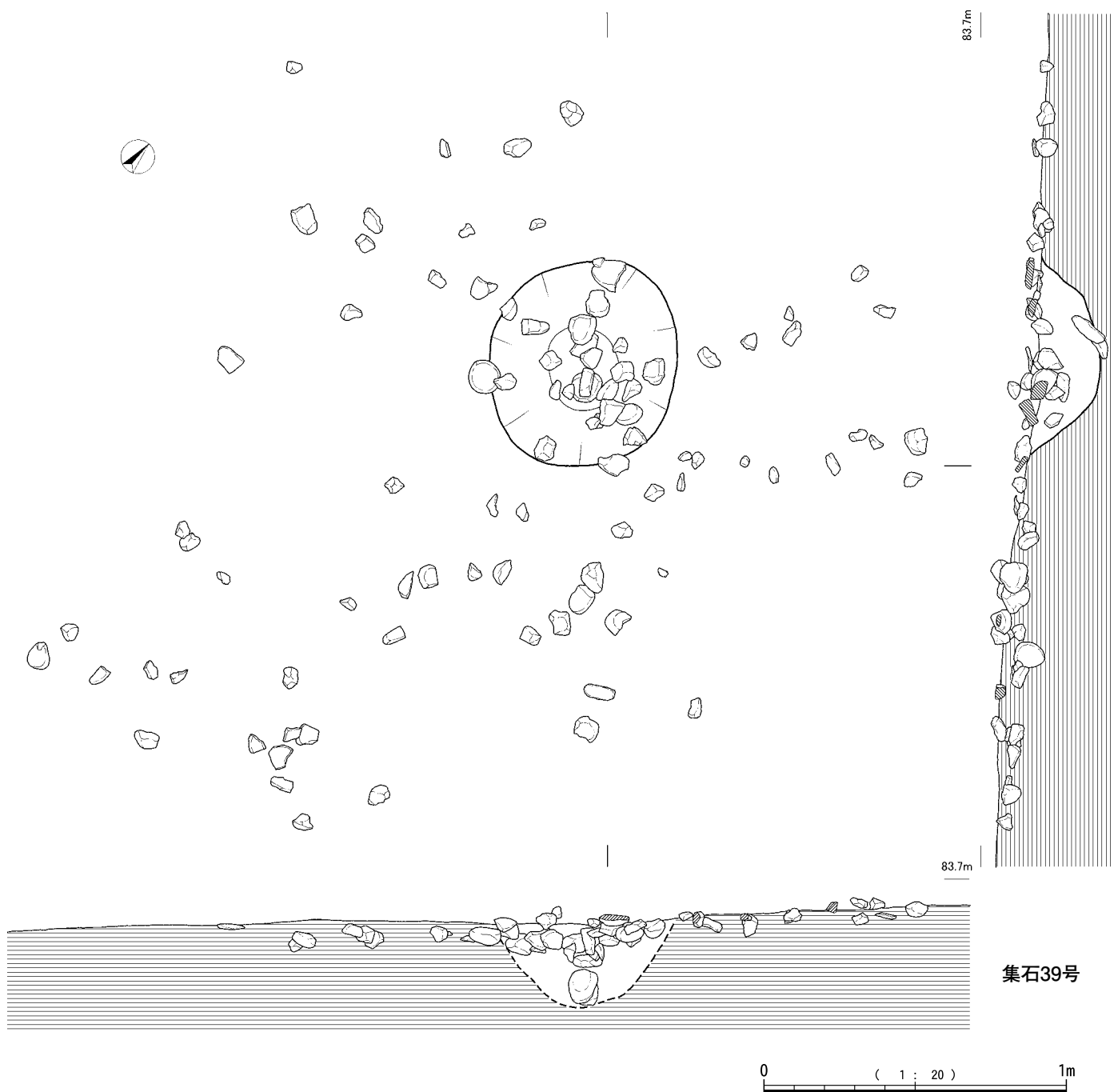
第60図 集石39号
