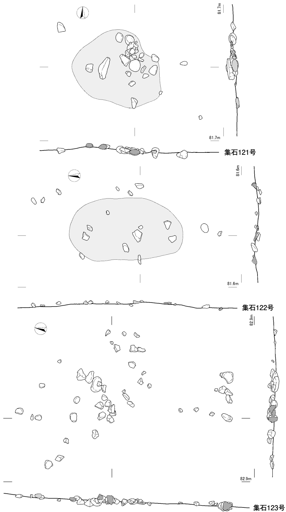
第84図 集石121 ~ 123号
