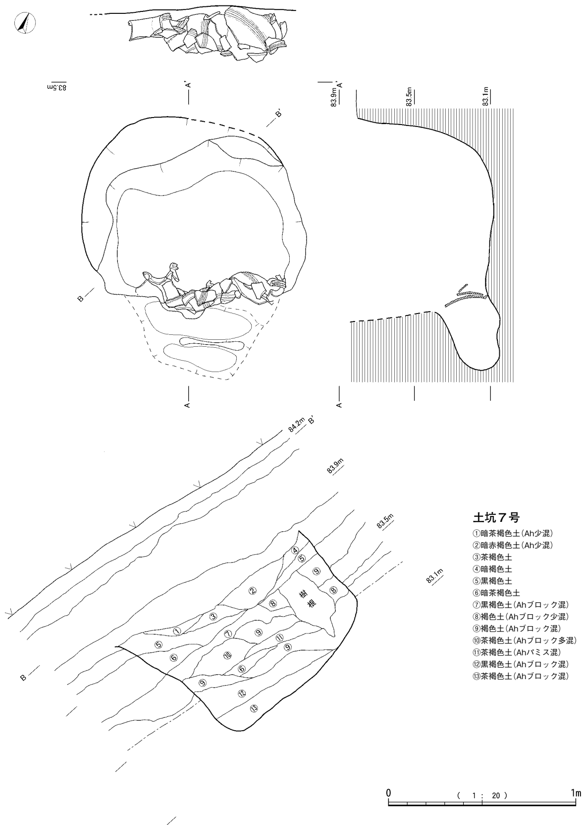
第236図 土坑7号
