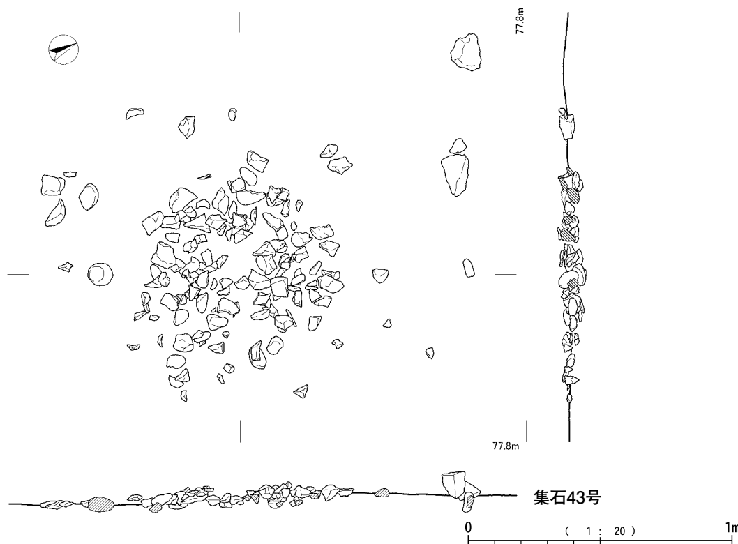
第62図 集石41～43号
