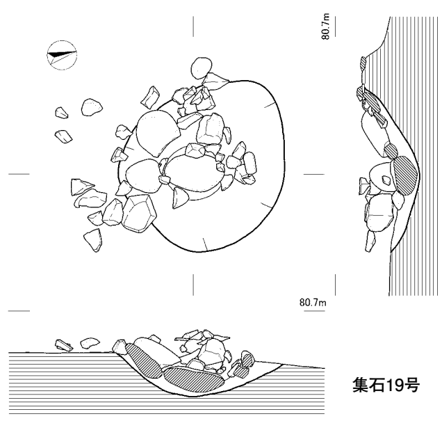
第52図 集石14～19号
