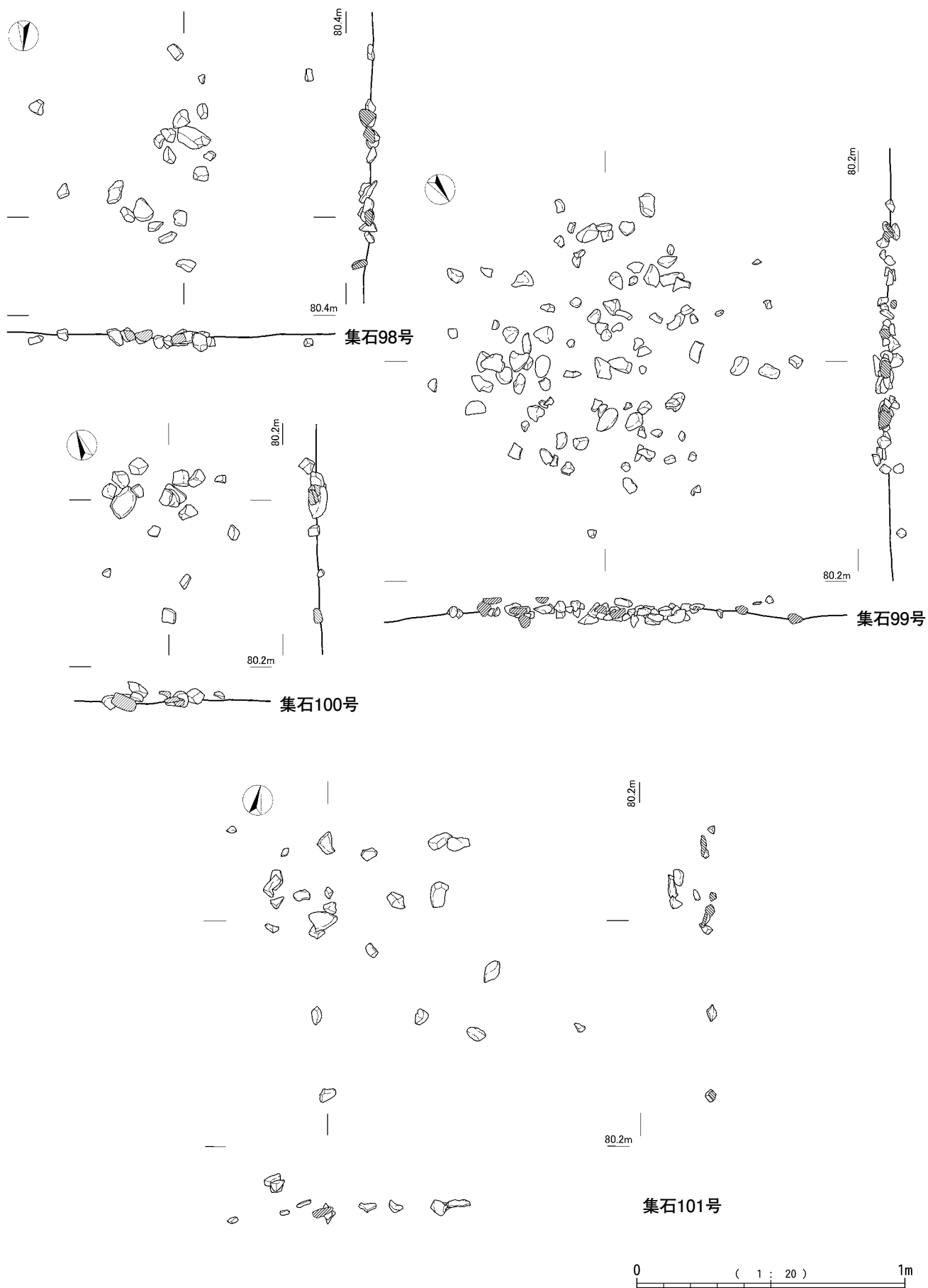
第77図 集石98 ~ 101号
