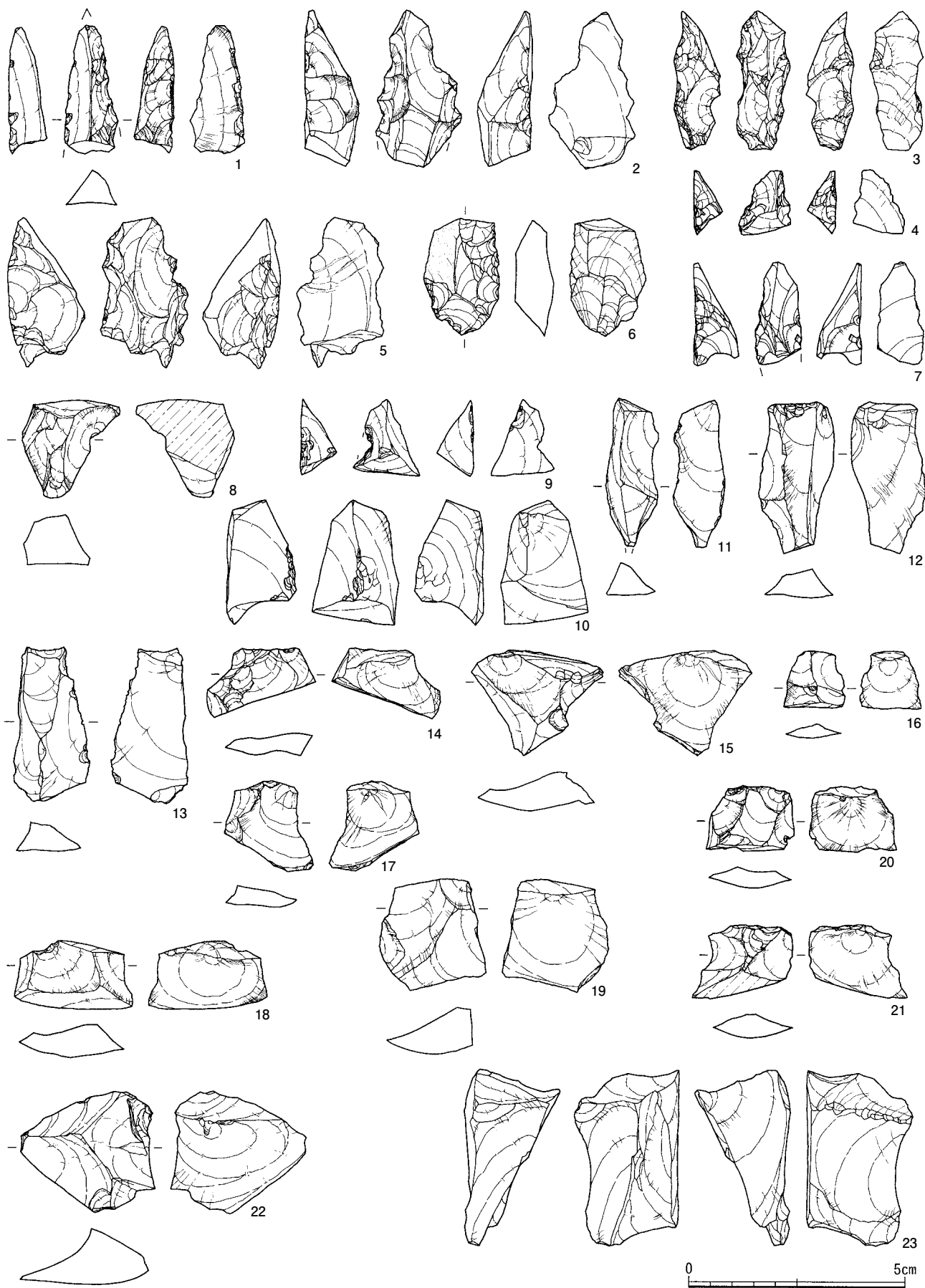
第36図 旧石器時代の石器（1）
