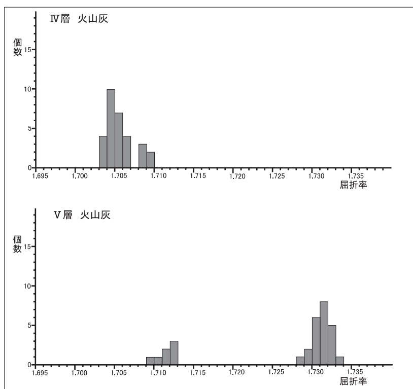
図3 斜方輝石の屈折率
