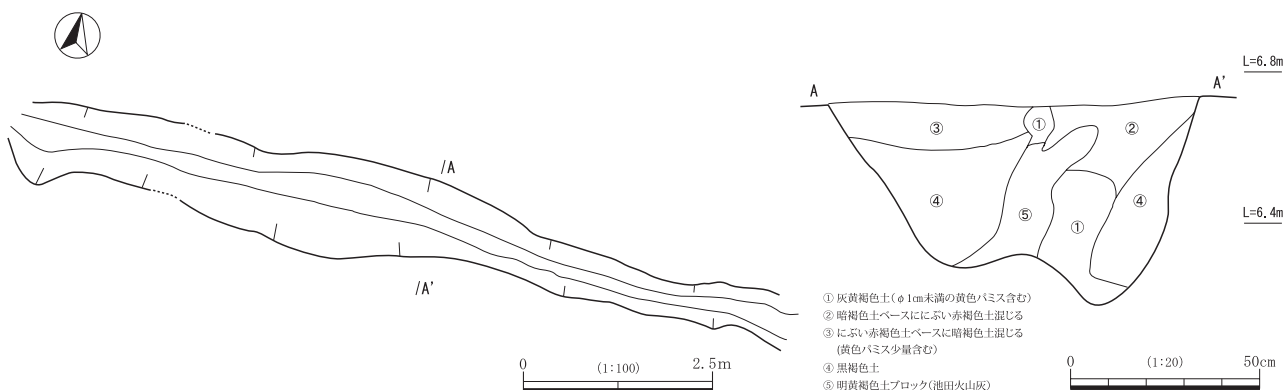
第4図 東区溝状遺構検出状況図
