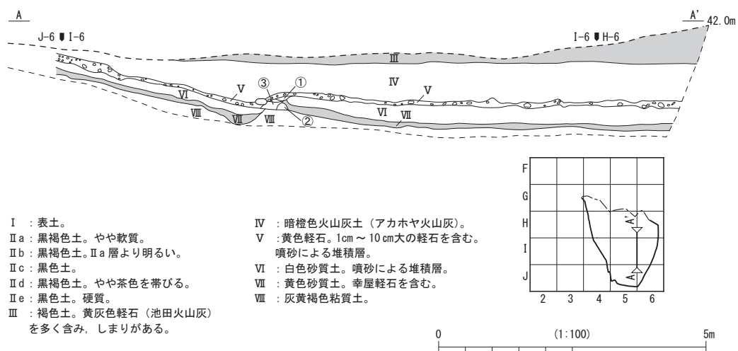
第4図 南北横断土層図
