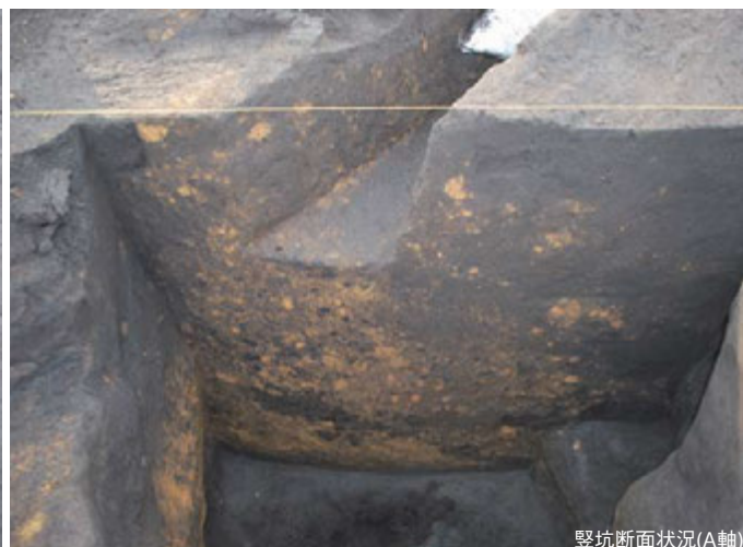
豎坑断面状況(A軸)
