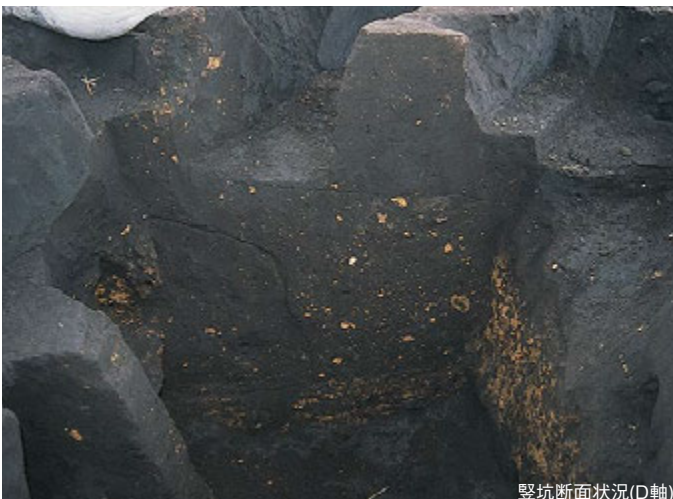
豎坑断面状況(D軸)
