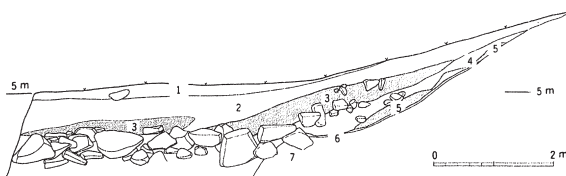
第2図 3トレンチ断面図
