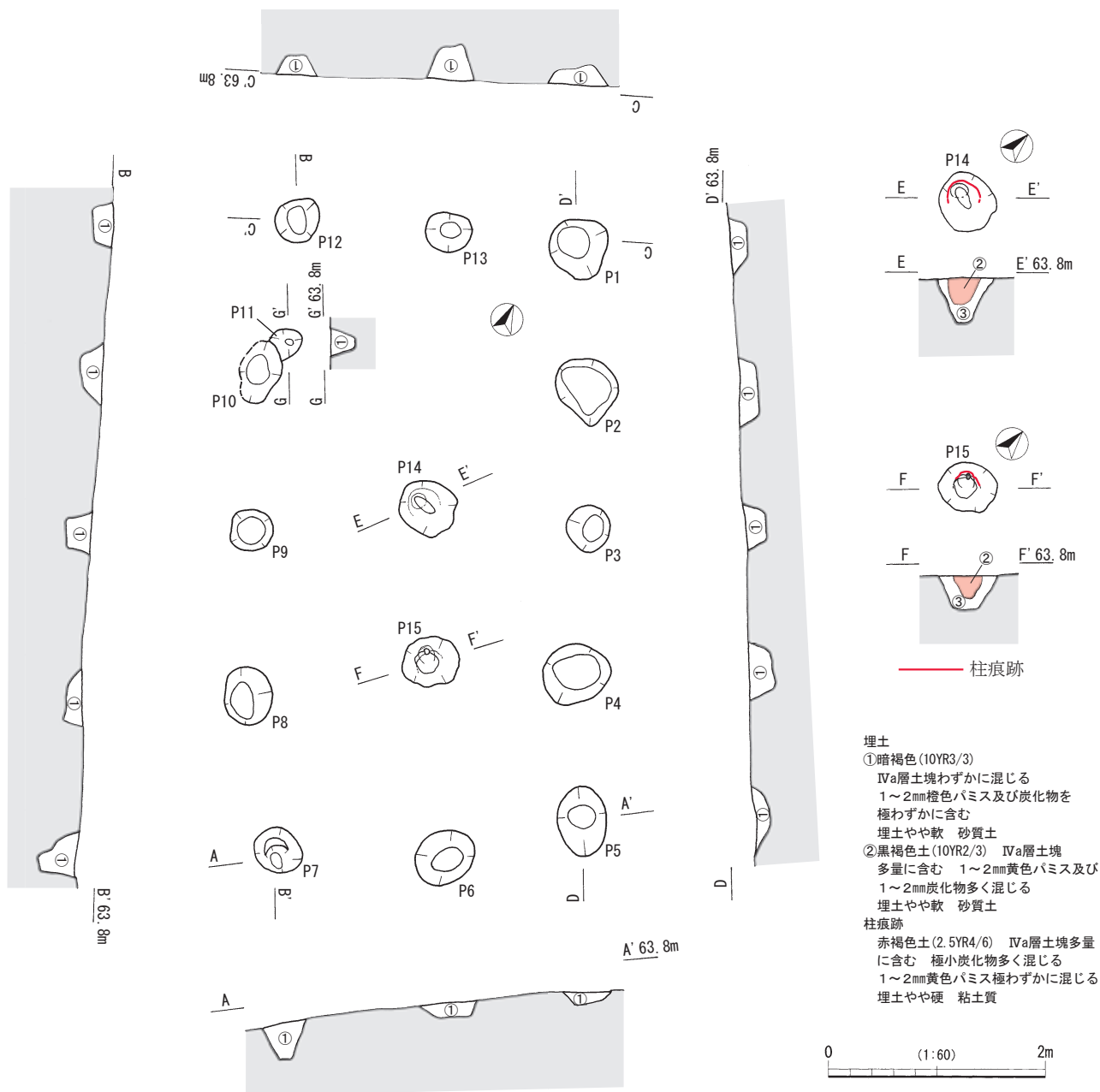
第12図 掘立柱建物跡1号
