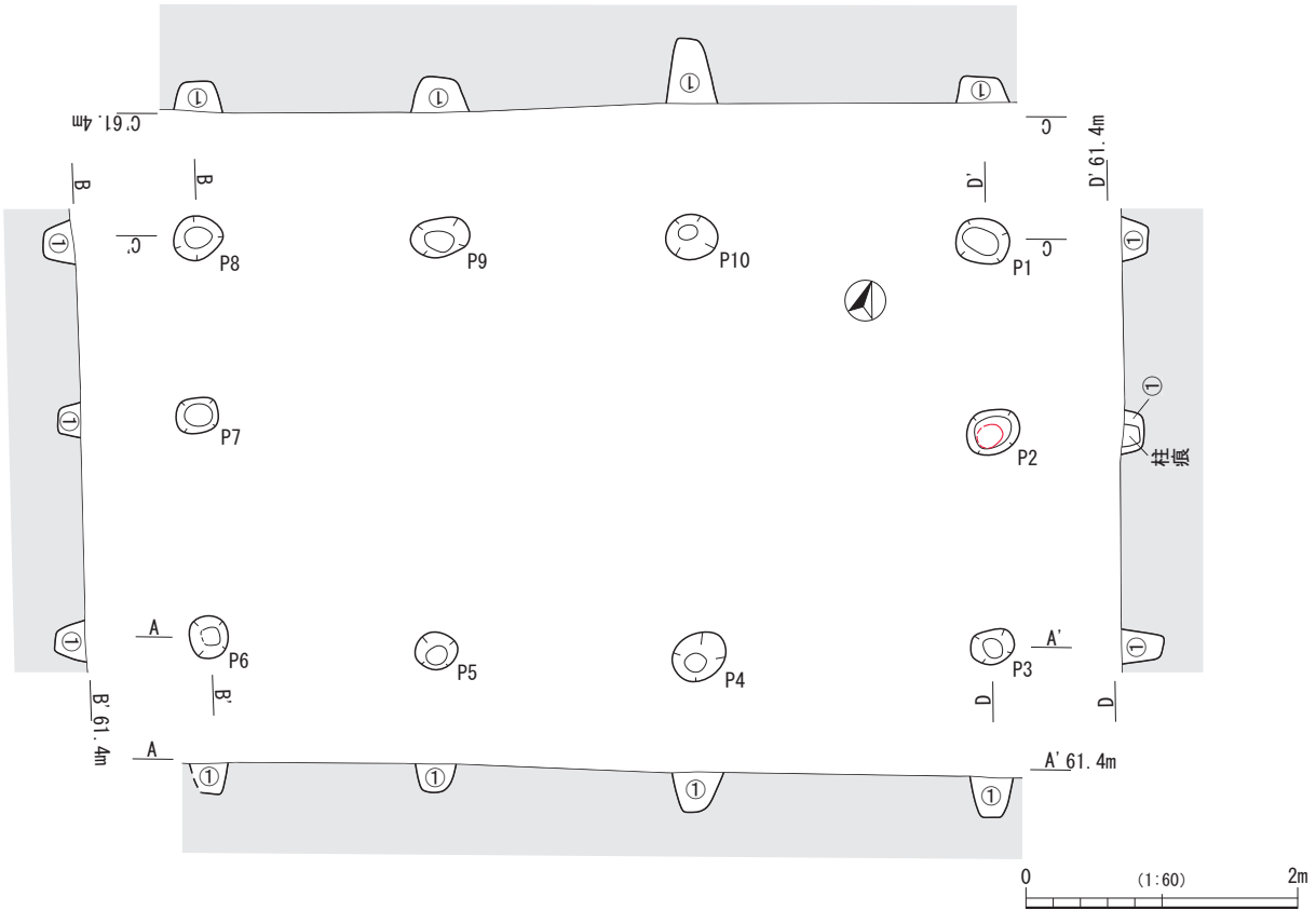
第 52 図 掘立柱建物跡 12・13 号
