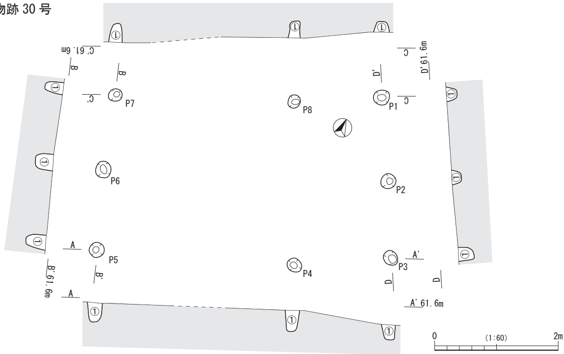
第 62 図 掘立柱建物跡 29・30 号
