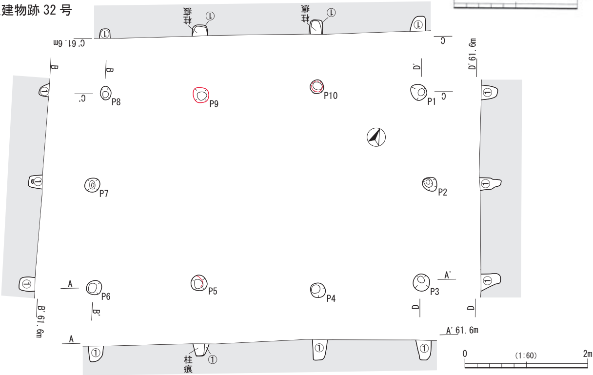
第 63 図 掘立柱建物跡 31・32 号
