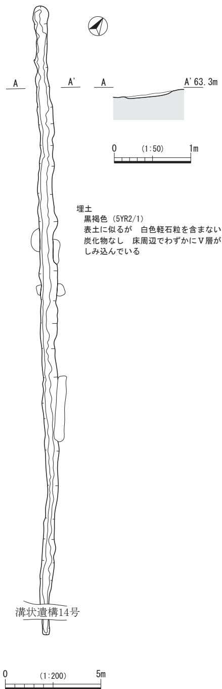
第 84 図 溝状遺構 12 号
