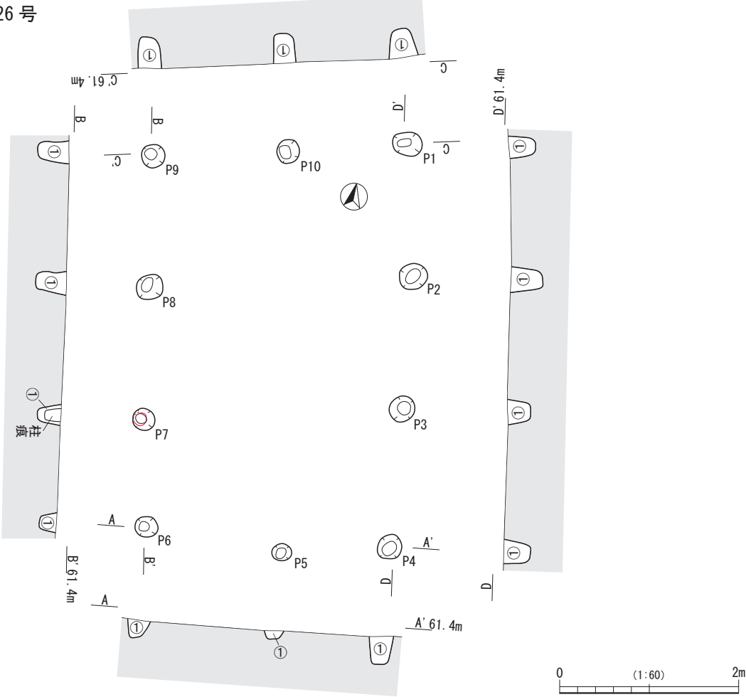
第 60 図 掘立柱建物跡 25・26 号
