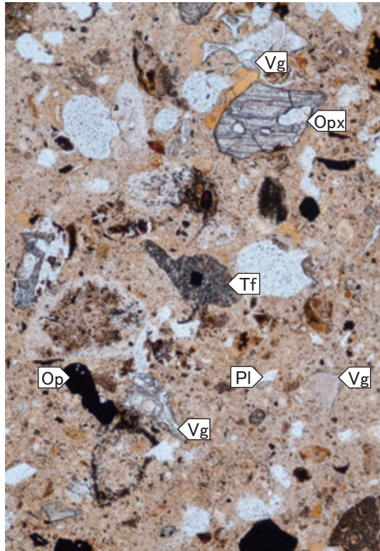
図版2 小牧遺跡の薄片
