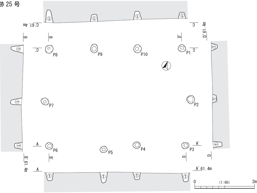
掘立柱建物跡 26 号
