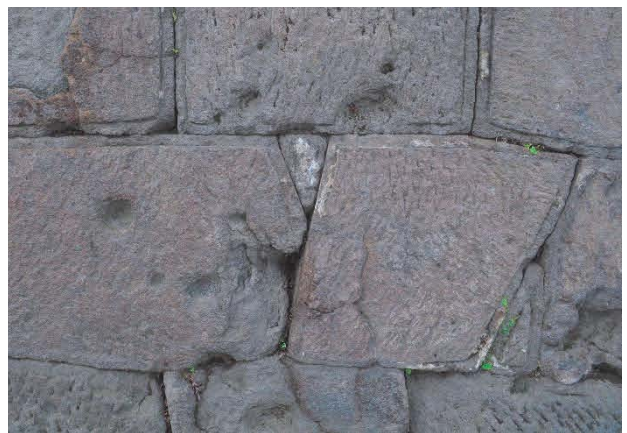
写真10 楔状詰石
