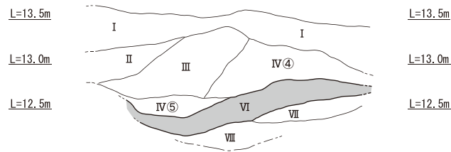
物原土層断面図②
