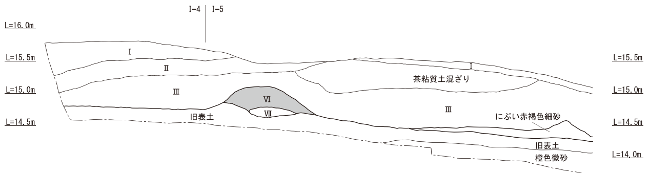
物原土層断面図②
