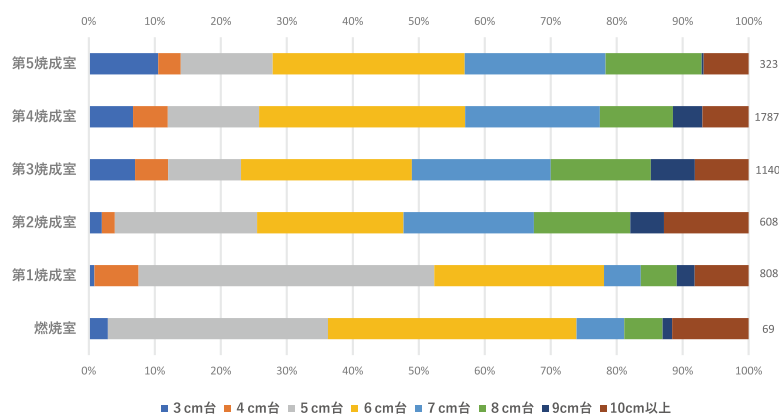
第110図 センベいの直径(1号窯各焼成室)
