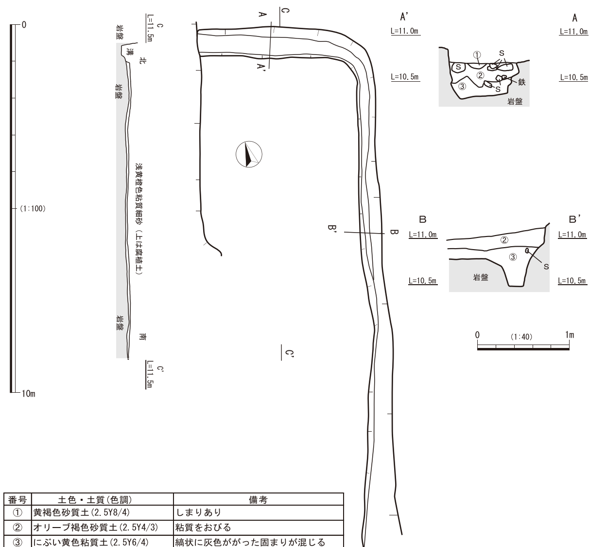
第32図 工房跡溝跡平面図, 土層断面図, 工房跡土層断面図
