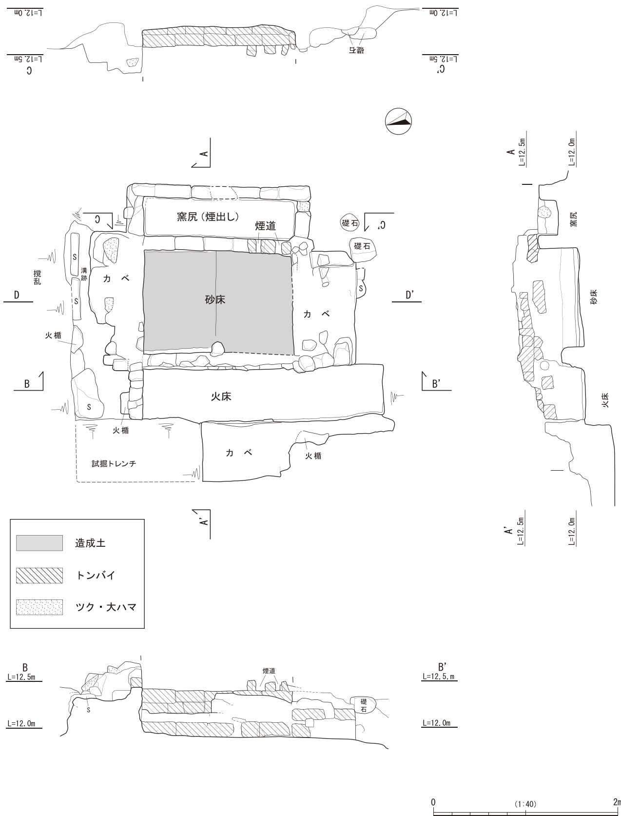
第21図 2号窯跡平面図及び見透し図
