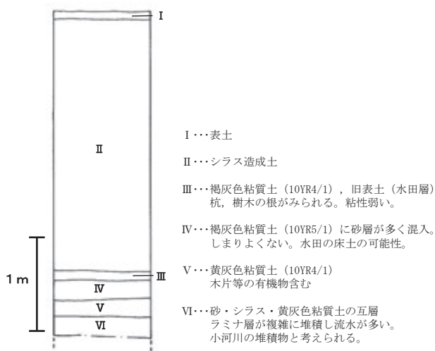
第74図 3TR土層 柱状模式図
